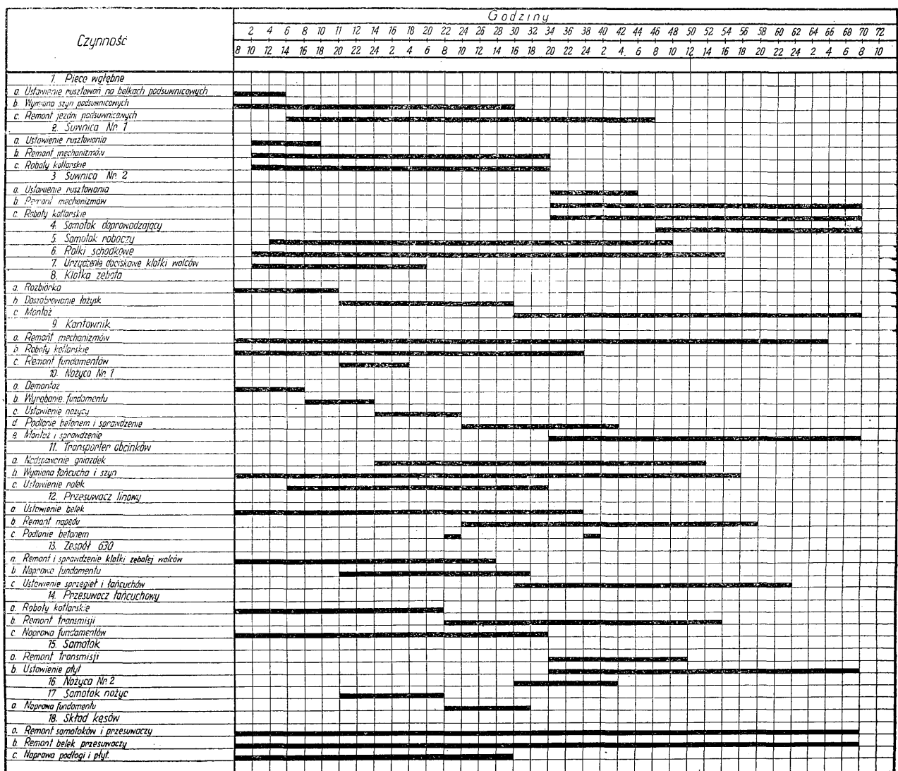
Rys. 5. Zbiorczy harmonogram naprawy zgniatacza
