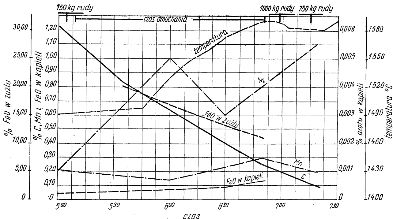
Rys. 5. Wykres przebiegu topu, do którego wdmuchiwało czysty azot (11)
