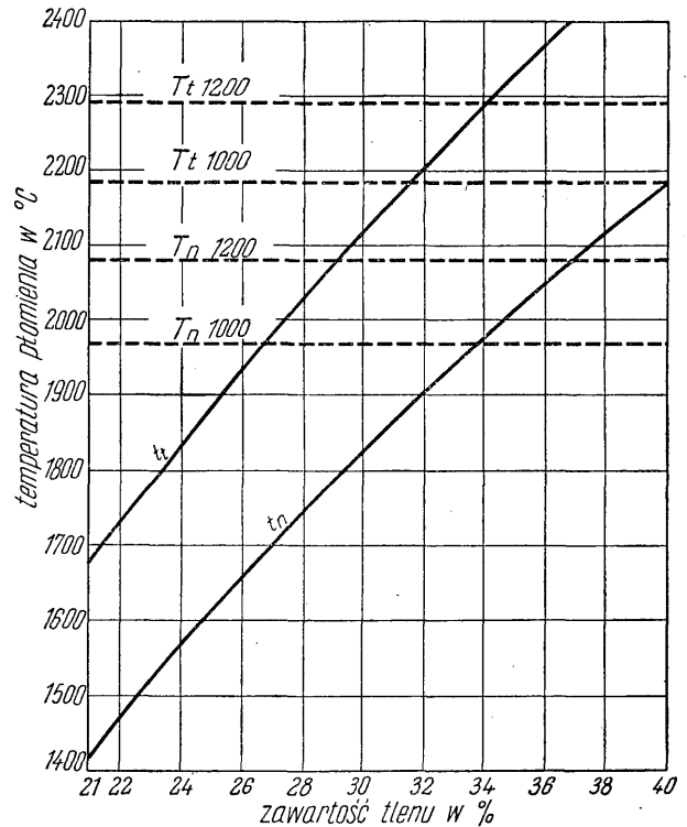
Rys. 1. Temperatura płomienia przy spalaniu gazu koksowego w zależności od zawartości tlenu w niepodgrzanym powietrzu do spalania: t_t — 2 teoretyczną ilością wzbogaconego powietrza t_n — 225% nadmiarem wzbogaconego powietrza, T_t 1000, T_t 1200 — temperatura płomienia przy spalaniu z teoretyczną ilością powietrza podgrzanego do 1000 i 1200 C (bez wzbogacenia w tlen) T_n 1000, T_n 1200 — jak poprzednio przy spalaniu z 25% nadmiarem powietrza
