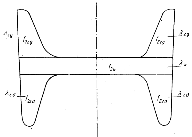
Rys. 8. Sposób podziału powierzchni wykroju dźwigara
