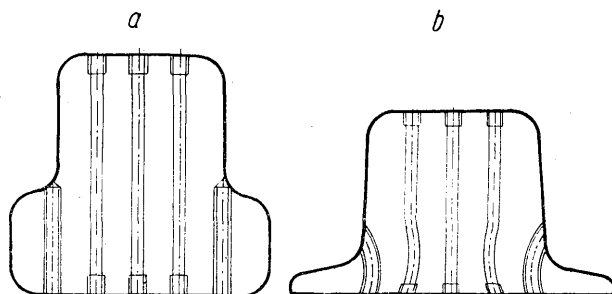
Rys. 6. Przekrój kęsiska: a — użytego do doświadczenia po przepuszczeniu w wykroju przedosadczym, b — przewalcowanego w wykroju osadczym
