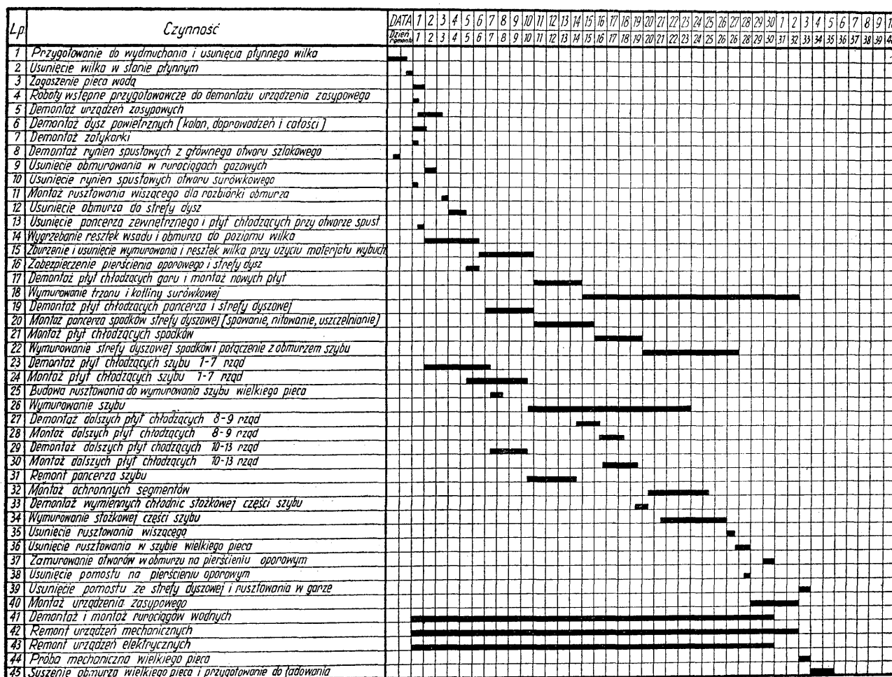
Rys. 2. Harmonogram kapitalnej naprawy wielkiego pieca
