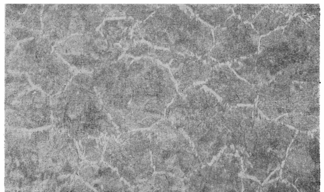
Rys. 13. Mikrostruktura części niehartowanej (ścianka i stopka) szyny z wytopu 2
