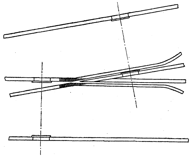
Rys. 14. Schemat rozjazdu kolejowego z zaznaczeniem najsilniej zużywających się części rozjazdu (miejsca zakreślowane)
