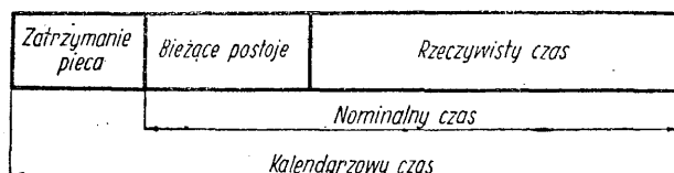
Rys. 1. Schemat podziału czasu służby wielkich pieców
