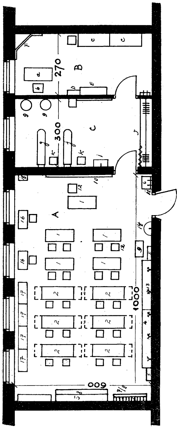
Rys. 4r. Plan sytuacyjny pracowni w szkołach żeńskich I : 100.
