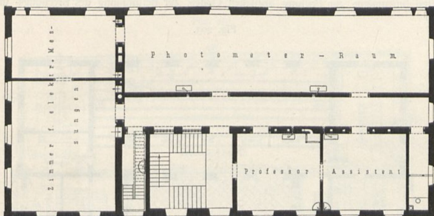
Obergeschoß.
