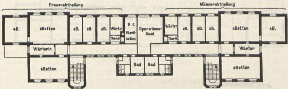
I. Obergehoß.
