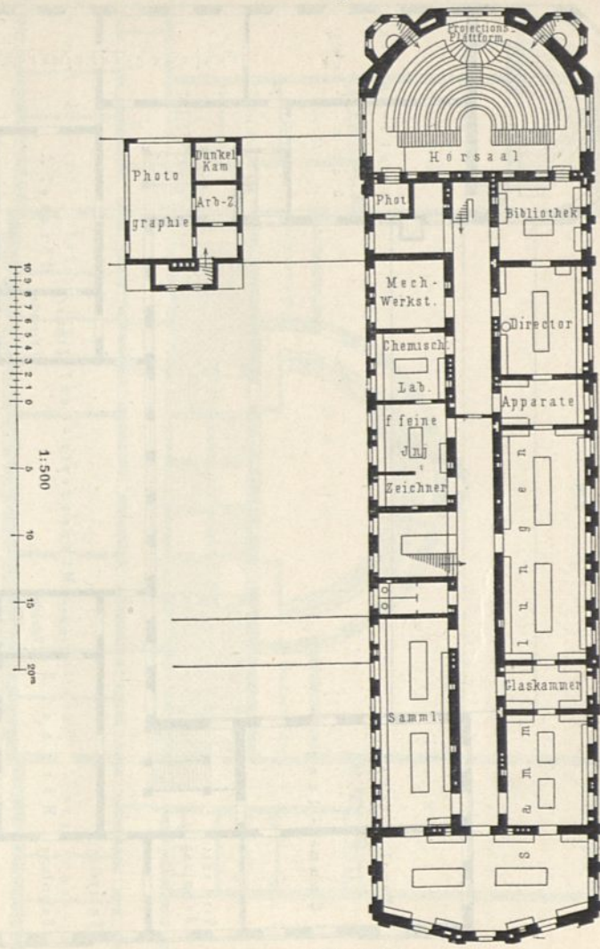
Obergeschoß.
