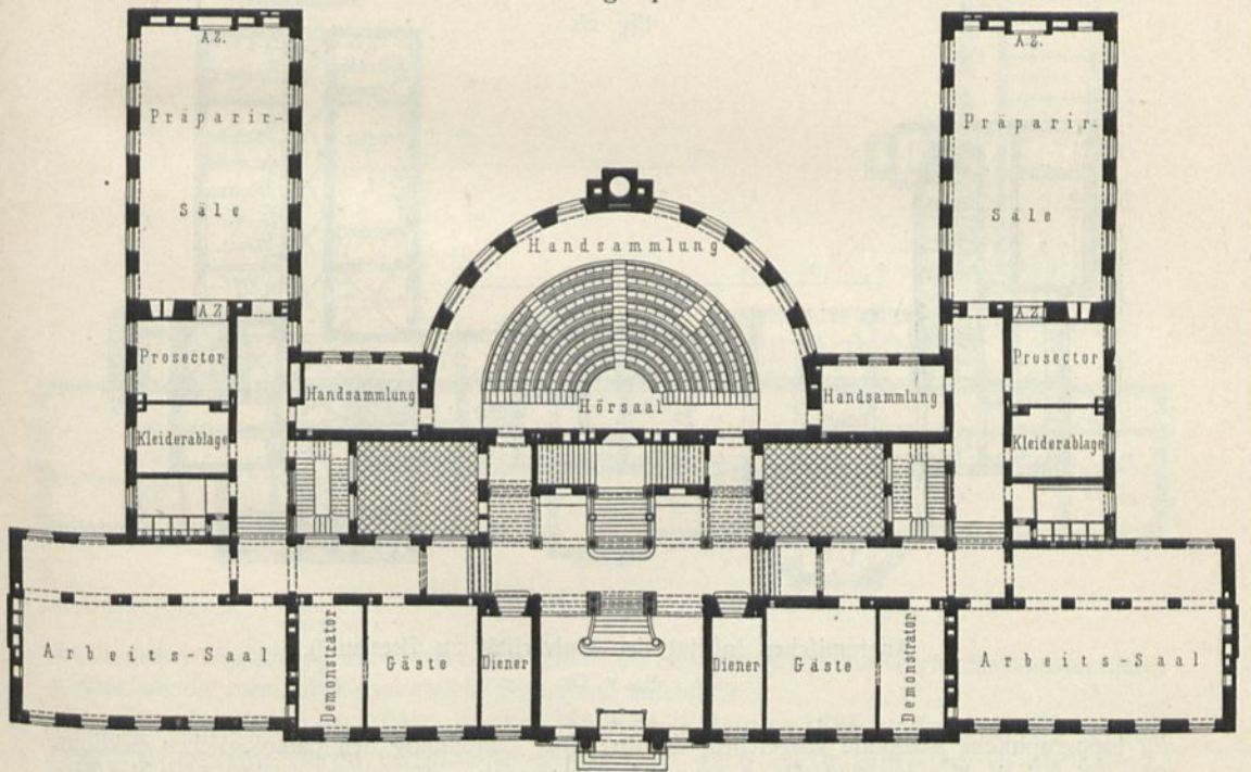
Erdgeschoß.
