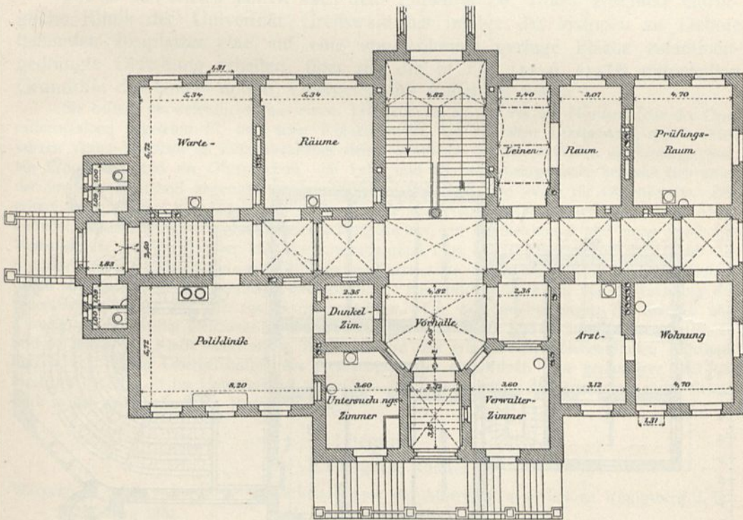
Erdgeschoß.
