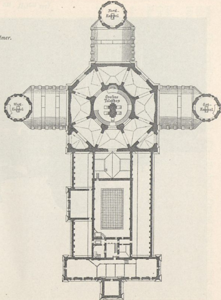
I. Obergeschoss.
