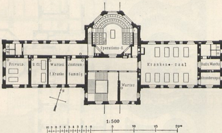
Chirurgische Klinik der Univerfität zu Heidelberg 60) .
