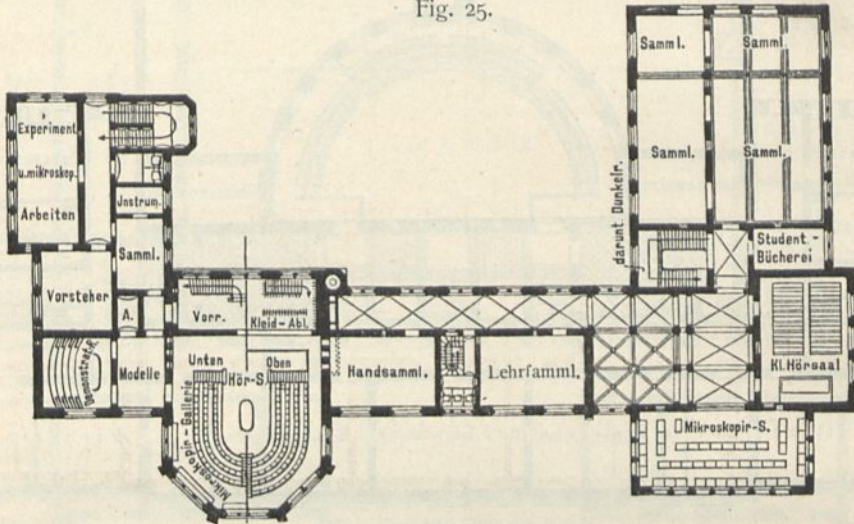
I. Obergechoß.
