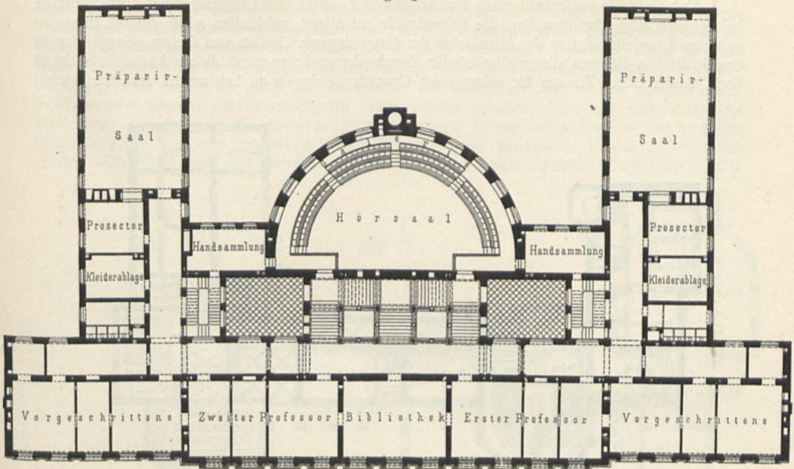
Obergeschoß.
