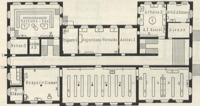
Erdgechoß.
