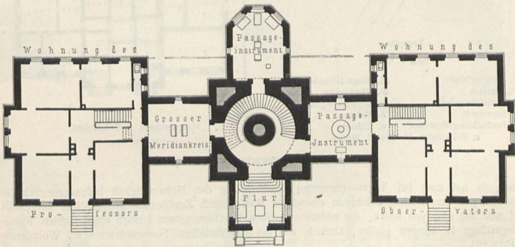
Erdgeschoß.
