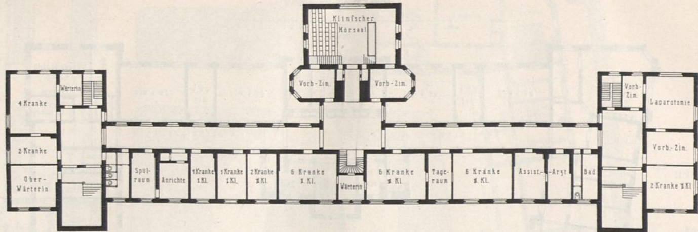
II. Obergechoß.
