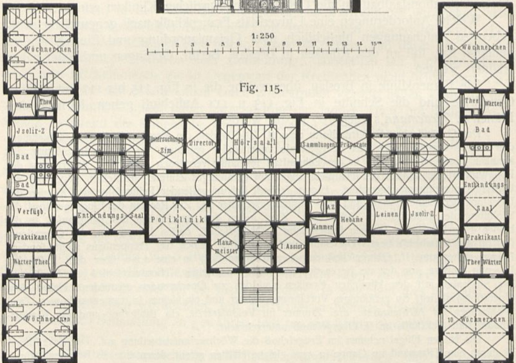
Erdgehoß.
