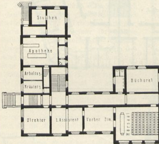
Erdgefchoß.
