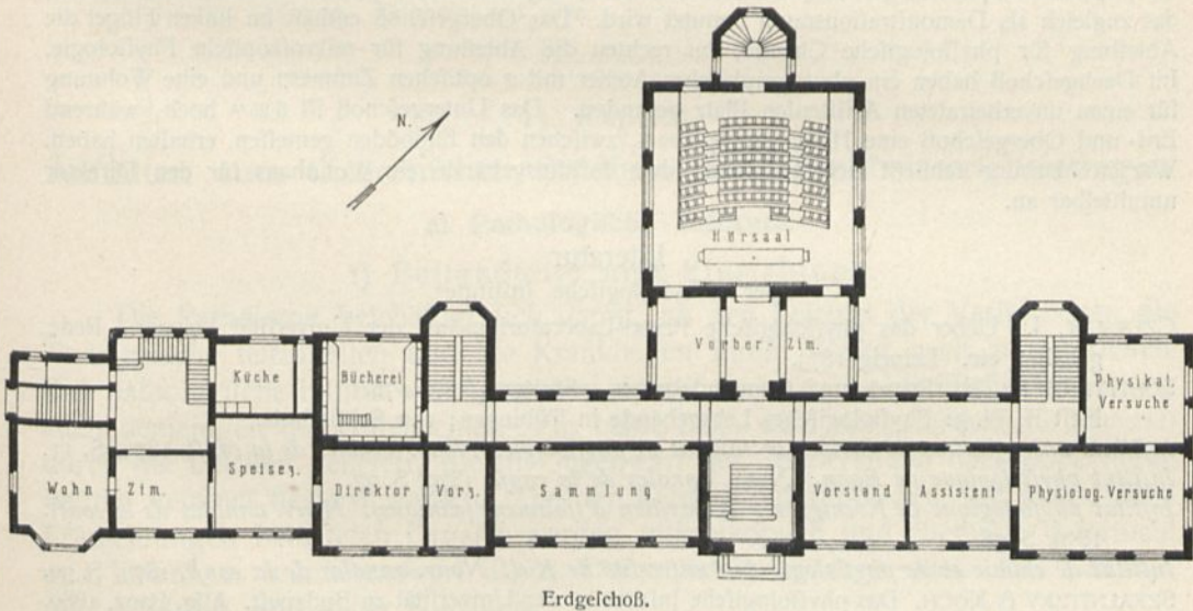
Erdgeschoß.
