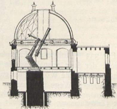
Lotrechter Schnitt 239) .
