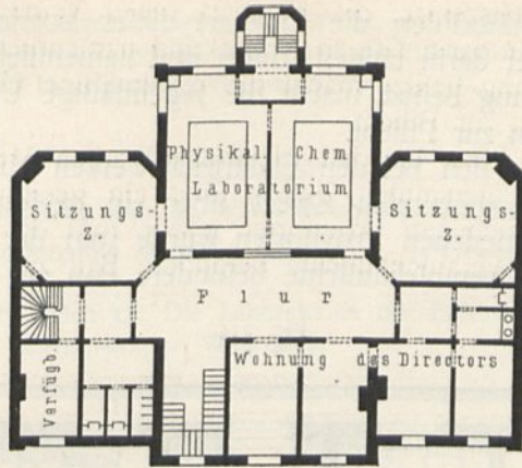
II. Obergechoß.
