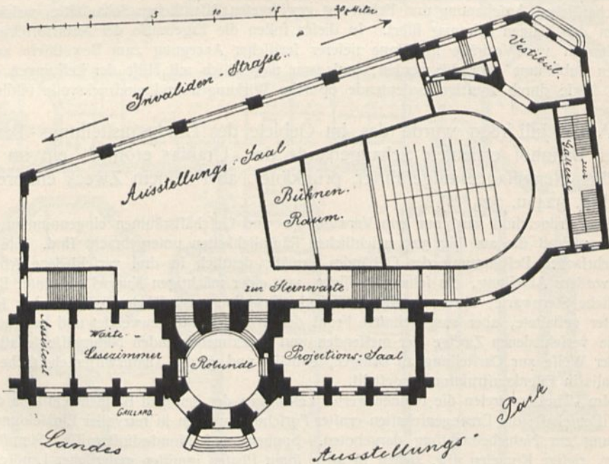
Obergehoß 325).
