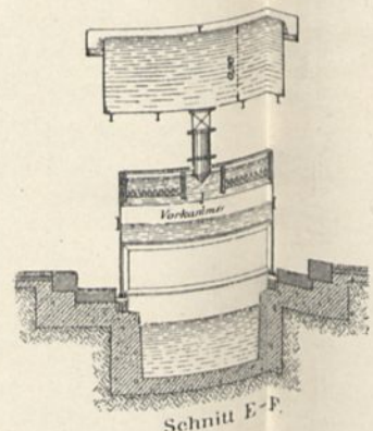
Schnitt E-F.
