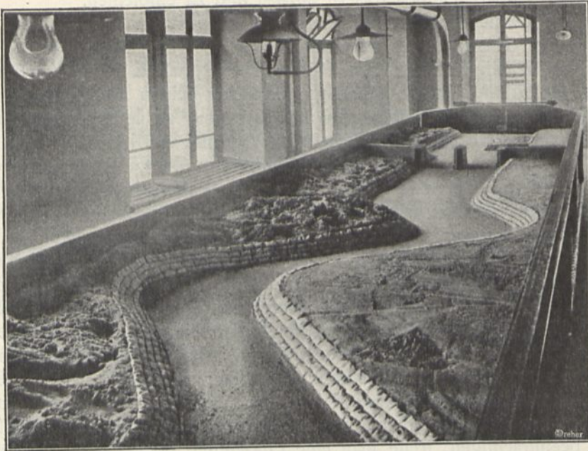
Blick in das Versuchserinne mit eingebautem Modellfluß. (Stromabwärts.)
