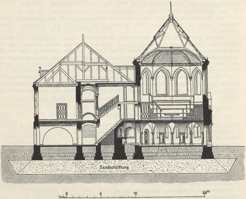
Querchnitt des Obduktionshauses nach AB.
