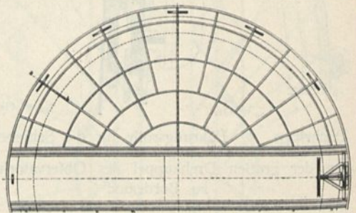
Rippenwerk der Drehkuppel der Sternwarte zu Göttingen 102) .
