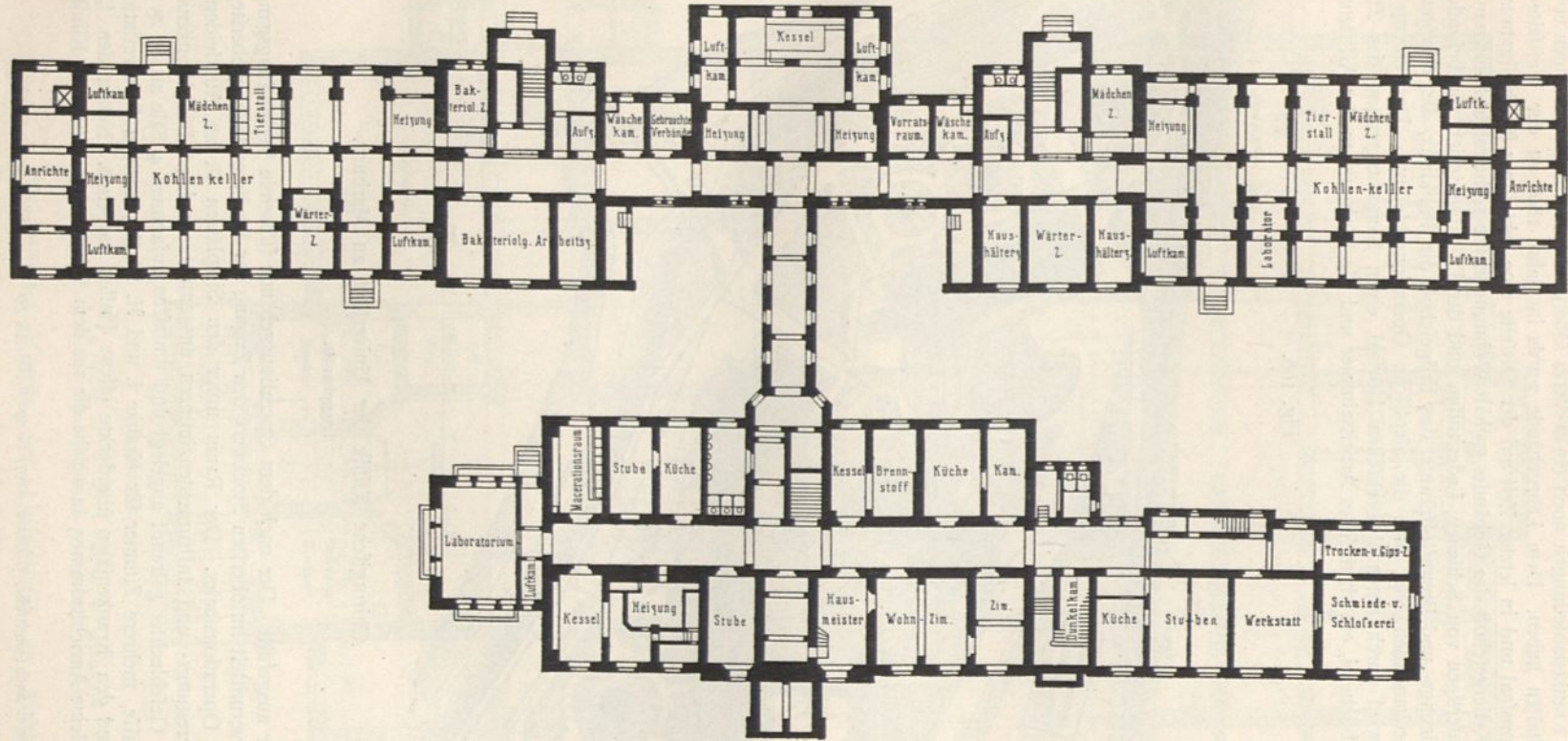
Kellergechoß.
