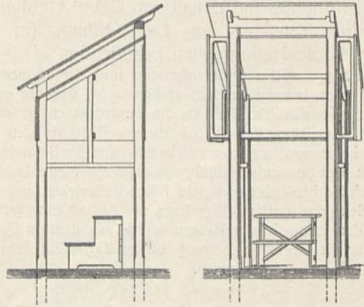
Französische Thermometerhütte.
