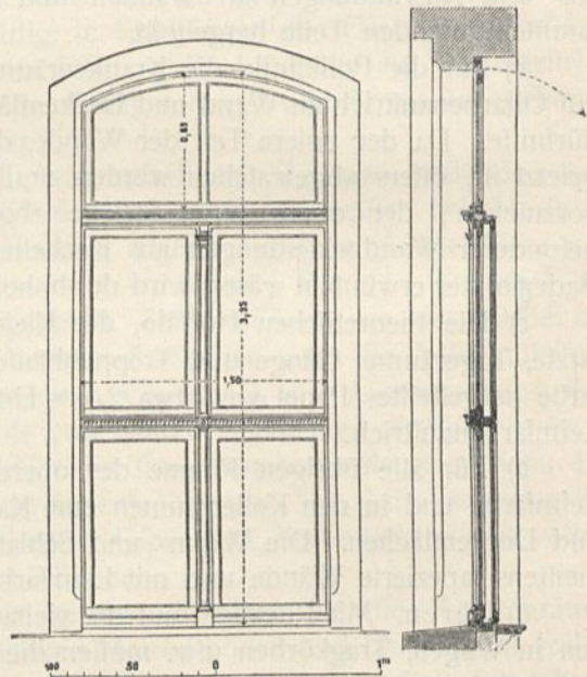
Fenster in der chirurgischen Klinik der Univerfität zu Bonn.
