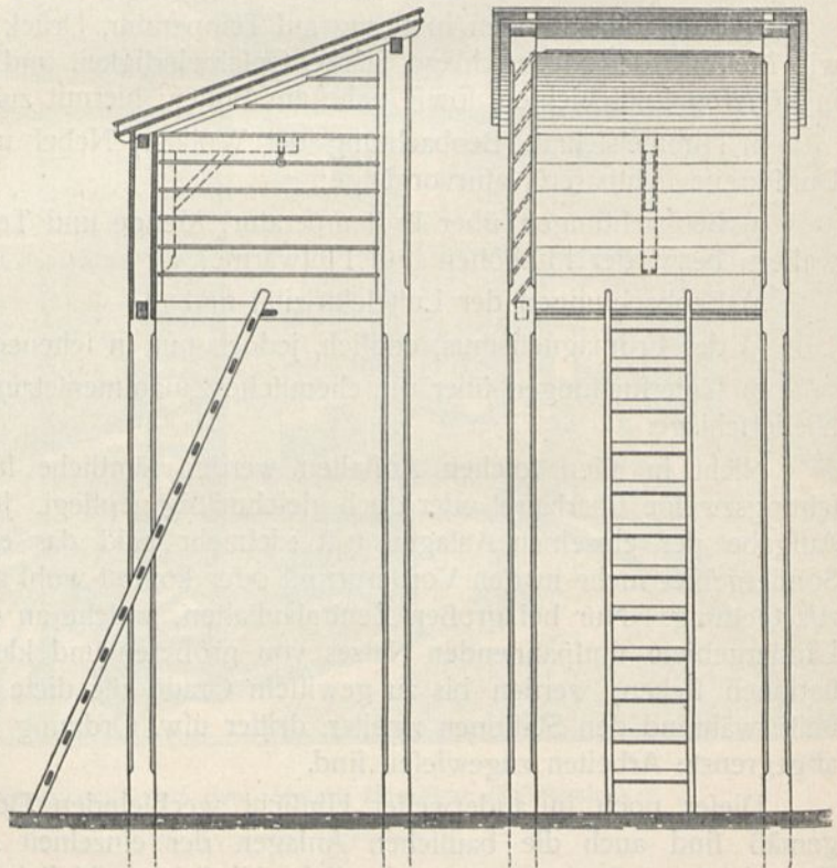
Wild'sche Thermometerhütte.
