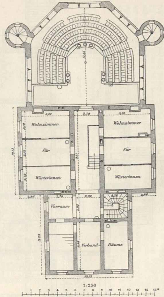
Obergeschoss.
