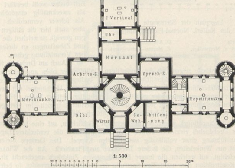
Universitäts-Sternwarte zu Bonn 215) .
