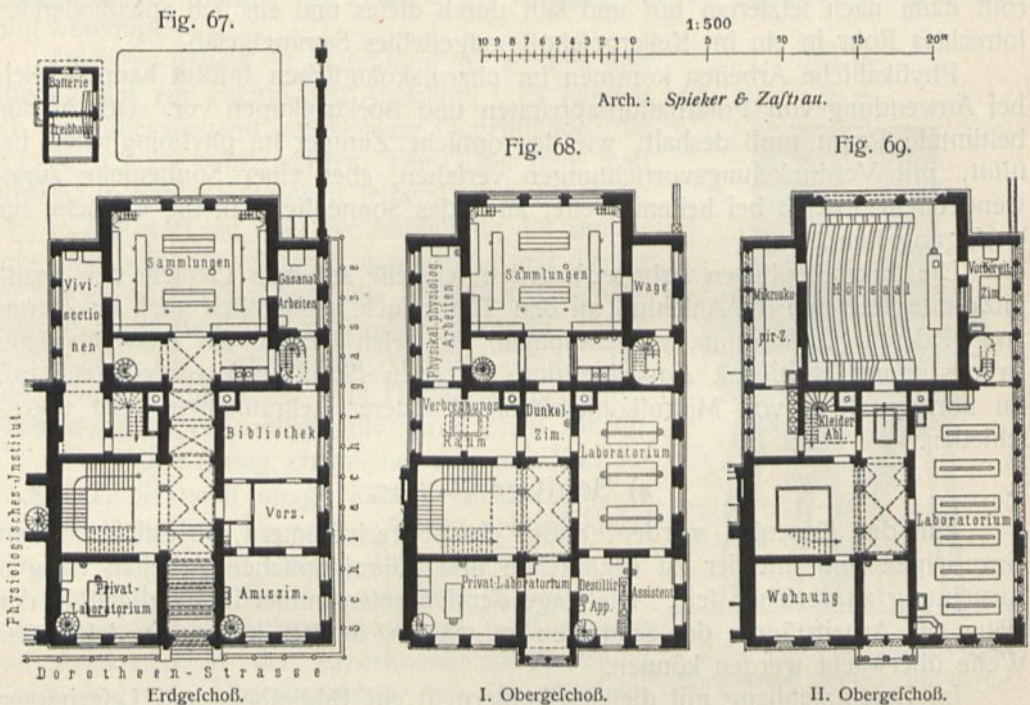
Pharmakologisches Institut der Universität zu Berlin.
