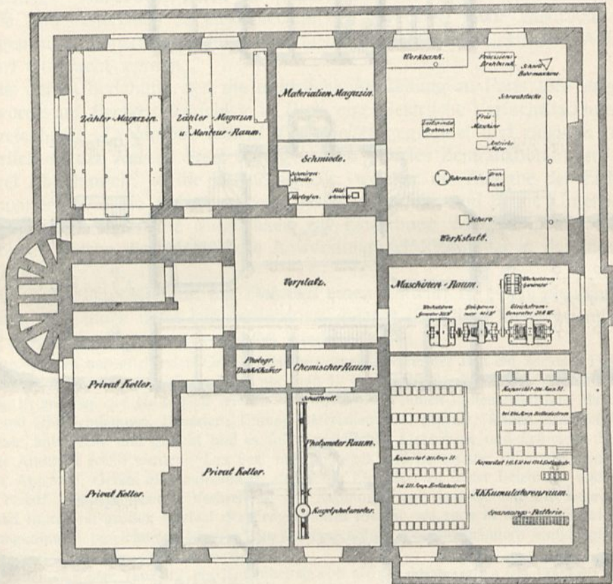
Sockelgechoß.
