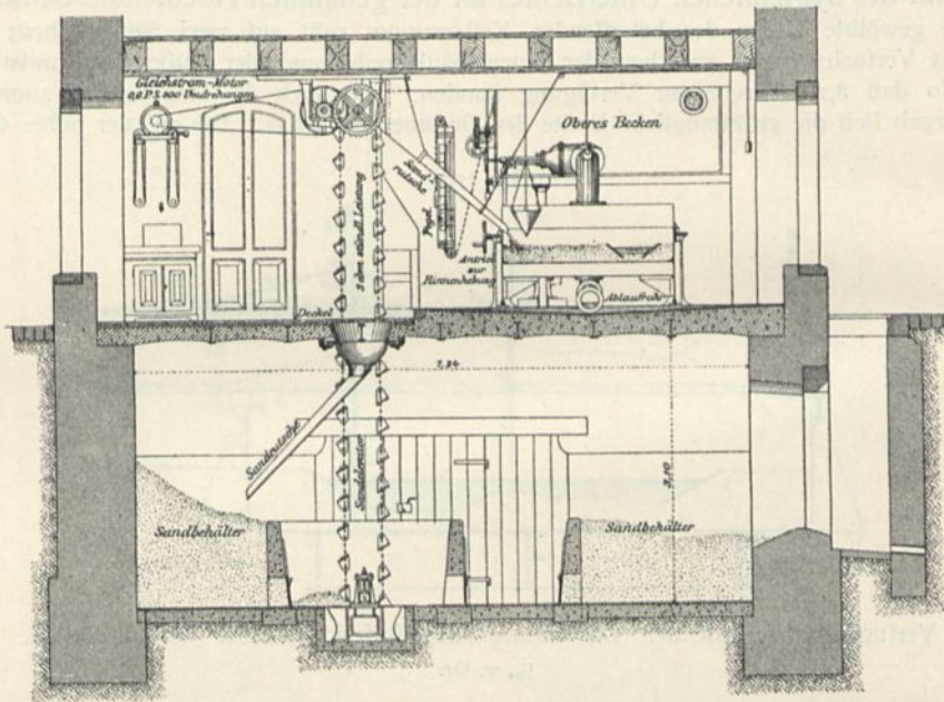
Querchnitt zur nebenstehenden Tafel 138) .
