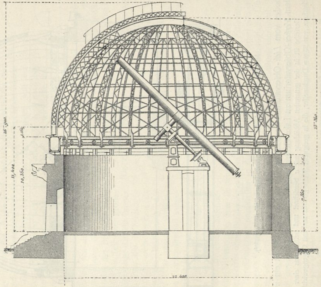
Querschnitt.
