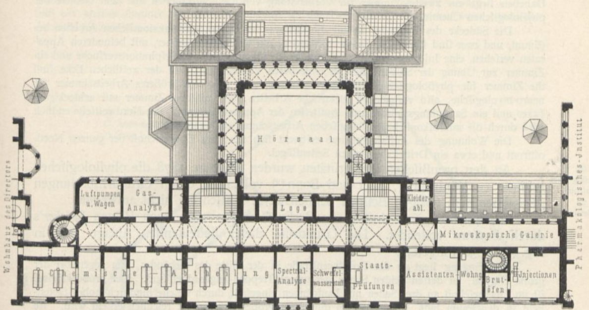
I. Obergechoß.
