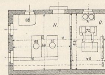
Maschinenhaus.
