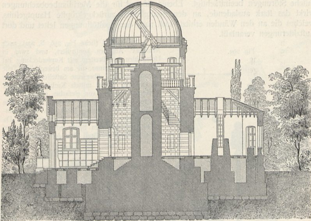
Querschnitt.
