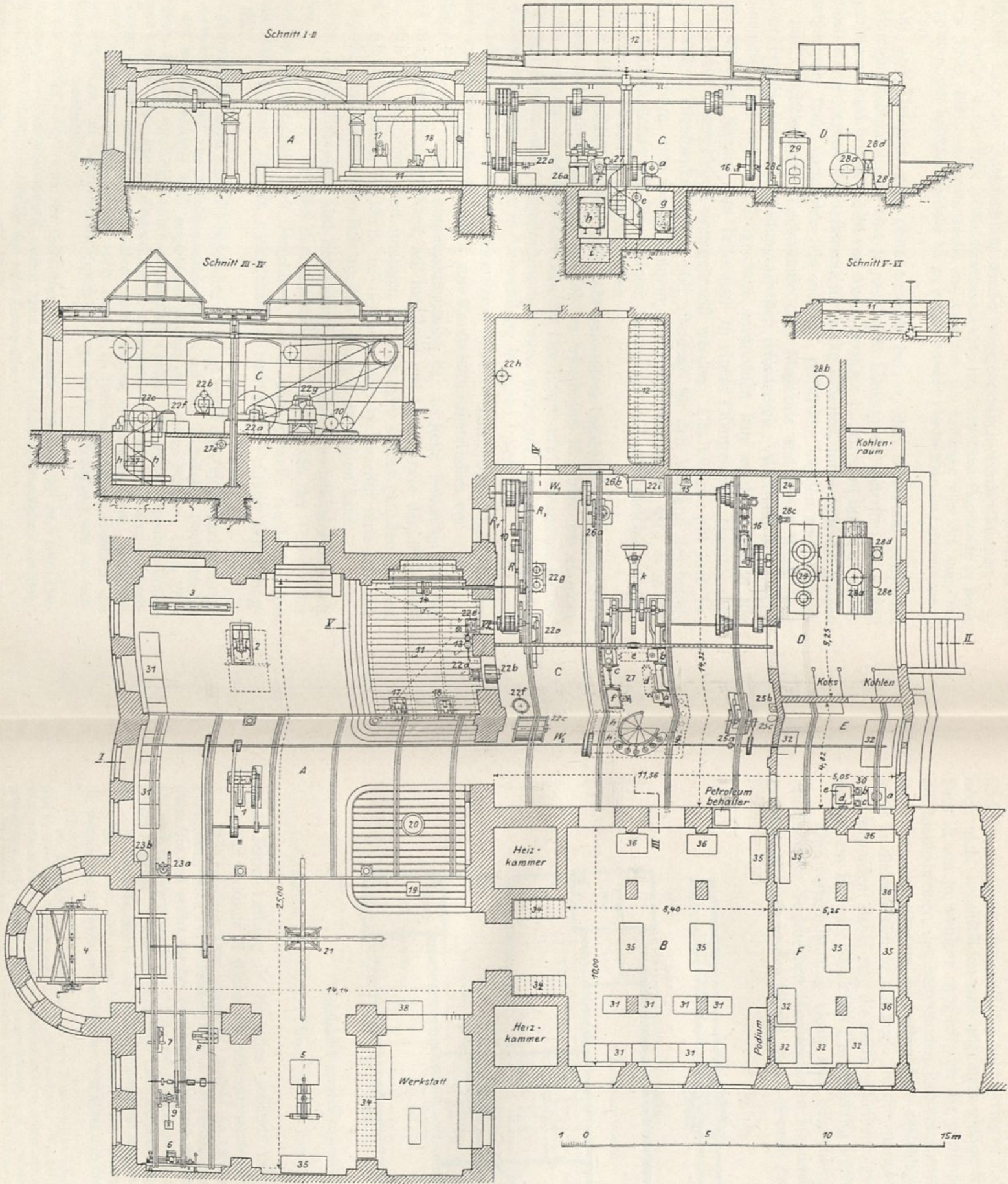
Ingenieurlaboratorium der Technischen Hochschule zu Hannover.
