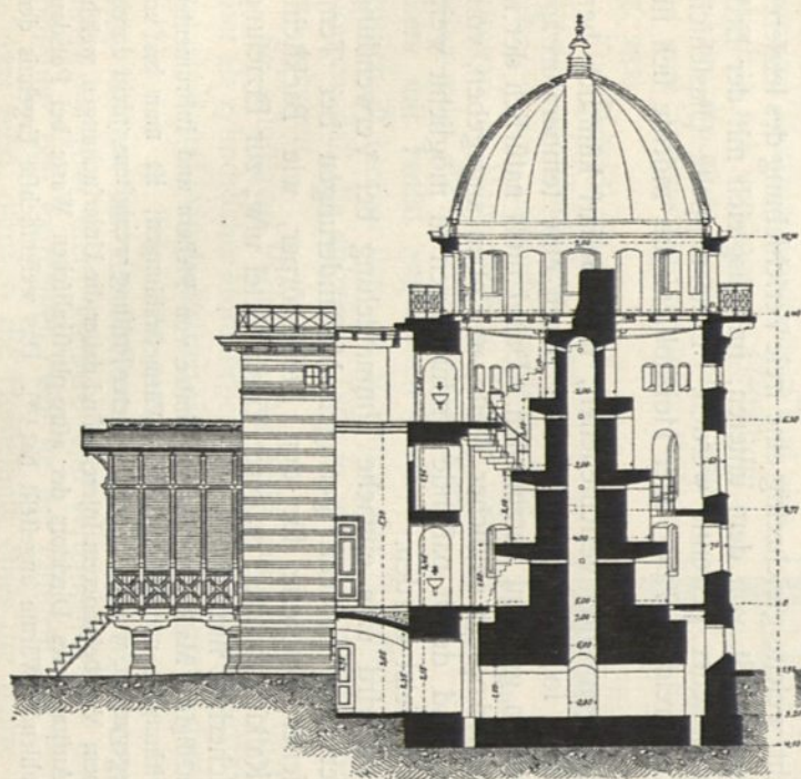
Westlicher Turm.
