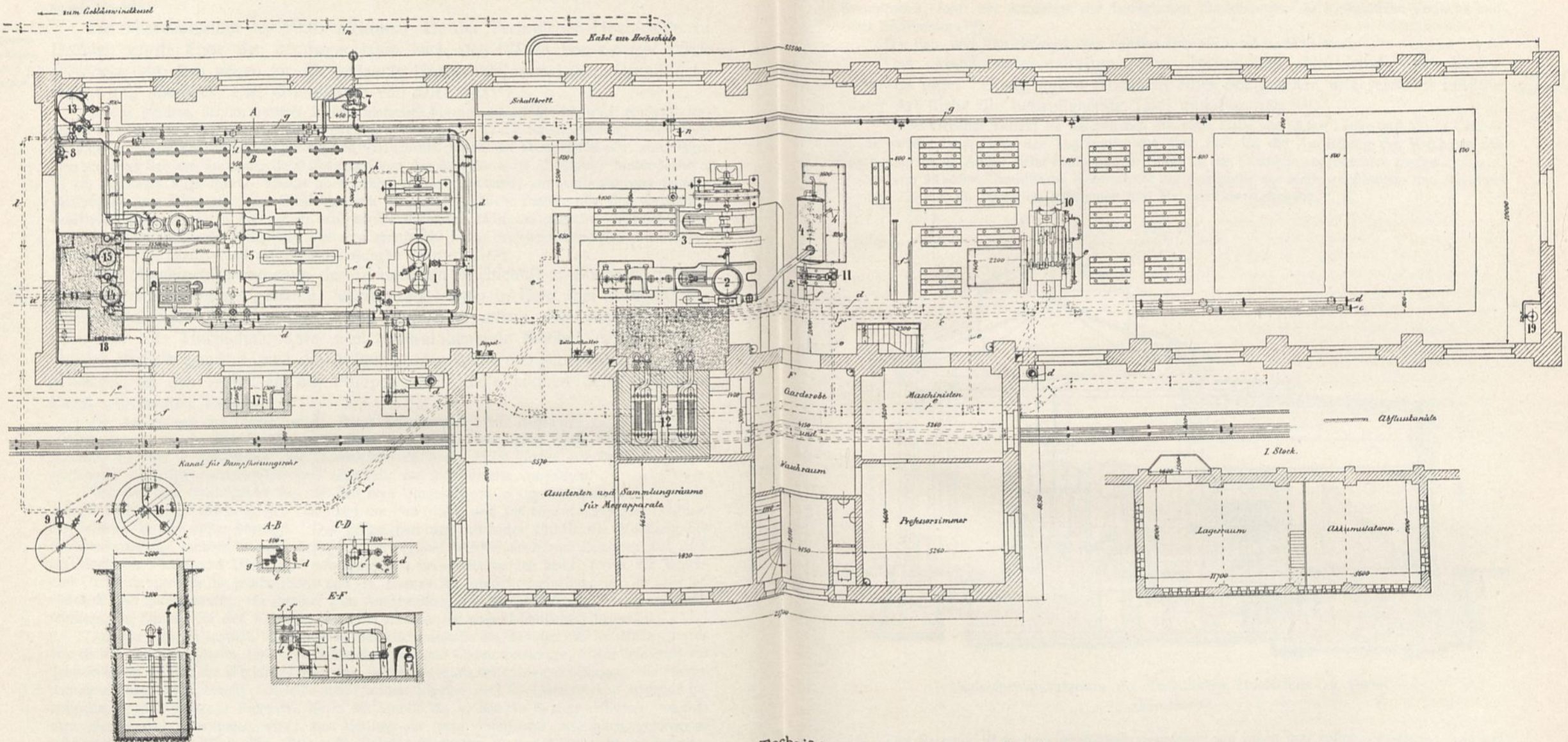
Maſchinenlaborium der Techniſchen Hochschule zu Berlin.
