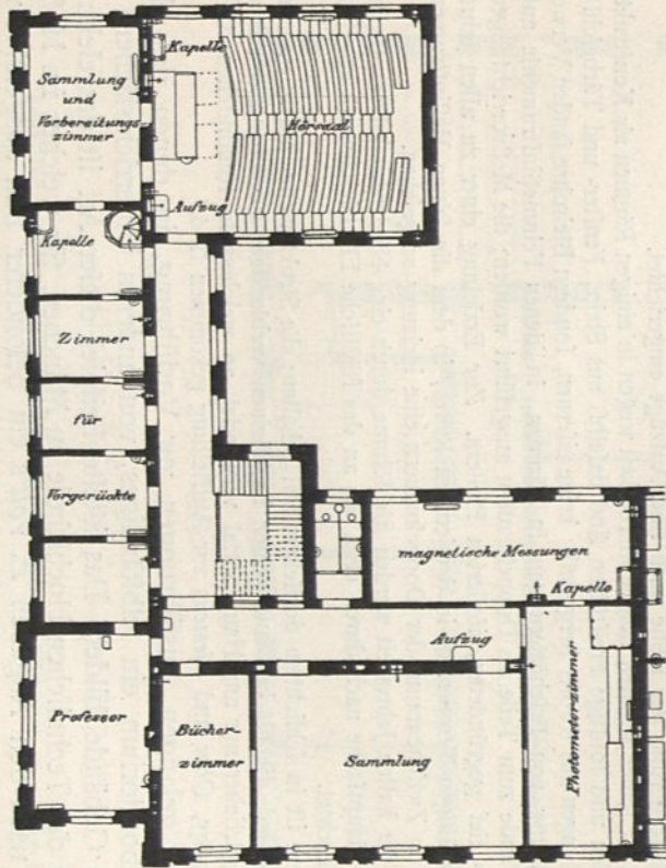
Erdgeschoß.
