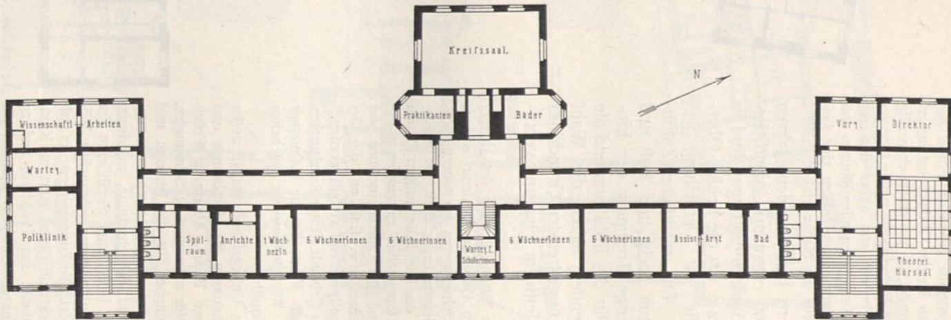
I. Obergechoß.
