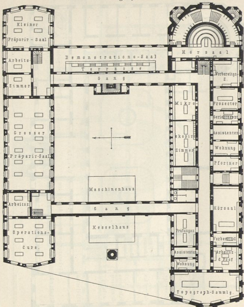
Erdgeschoß.
