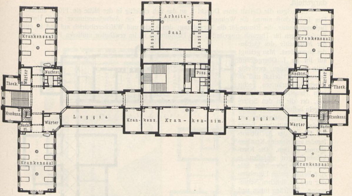
II. Obergeschoß.
