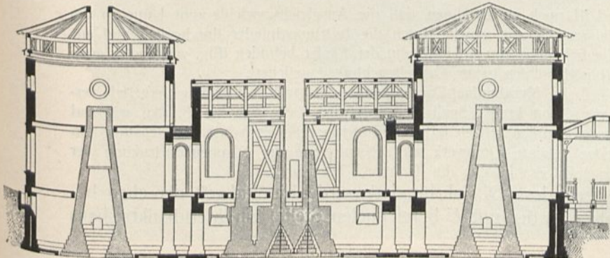
Längenschnitt.
