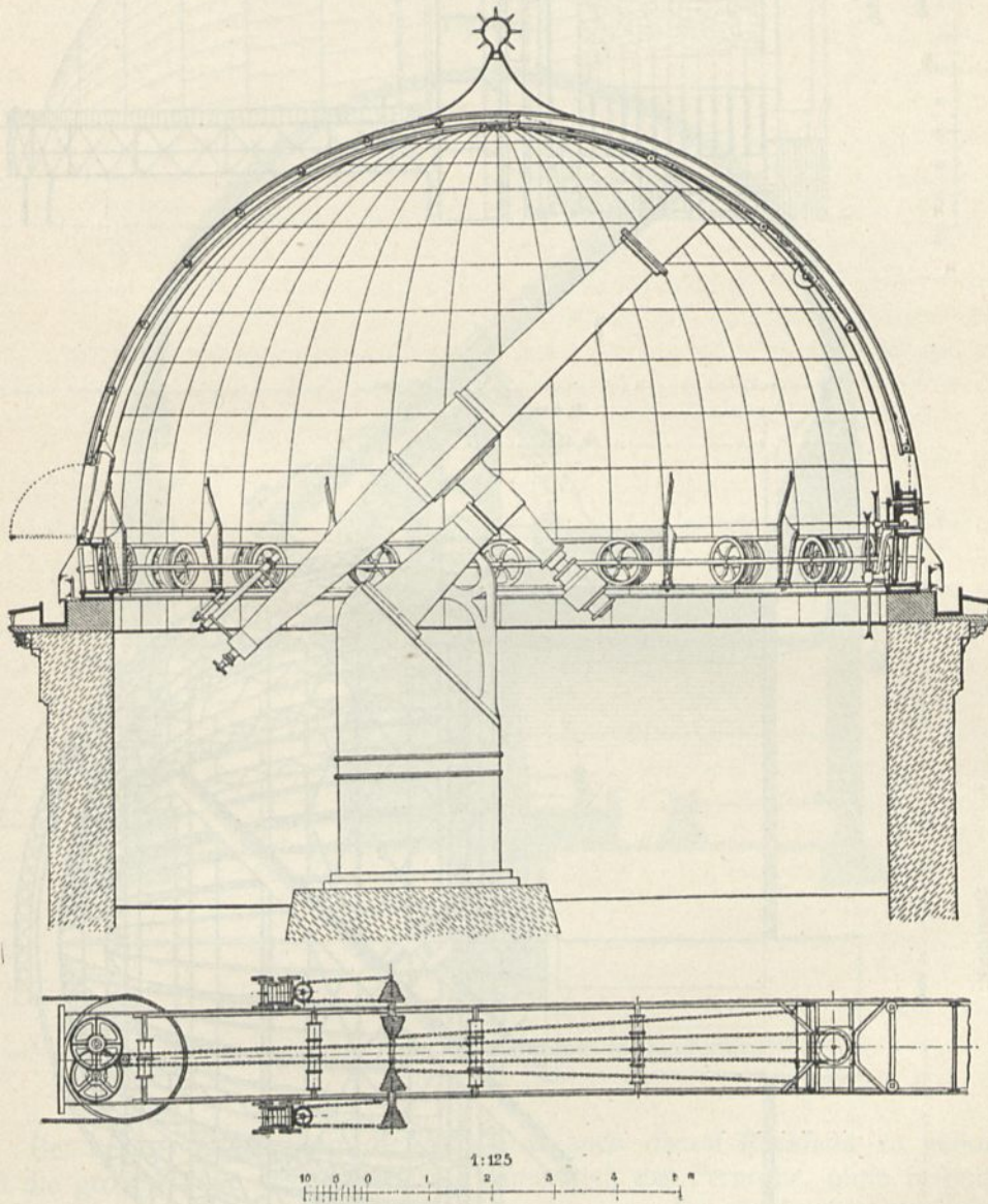
Mittlere Drehkuppel der Univerfitäts-Sternwarte zu Wien 185) .
