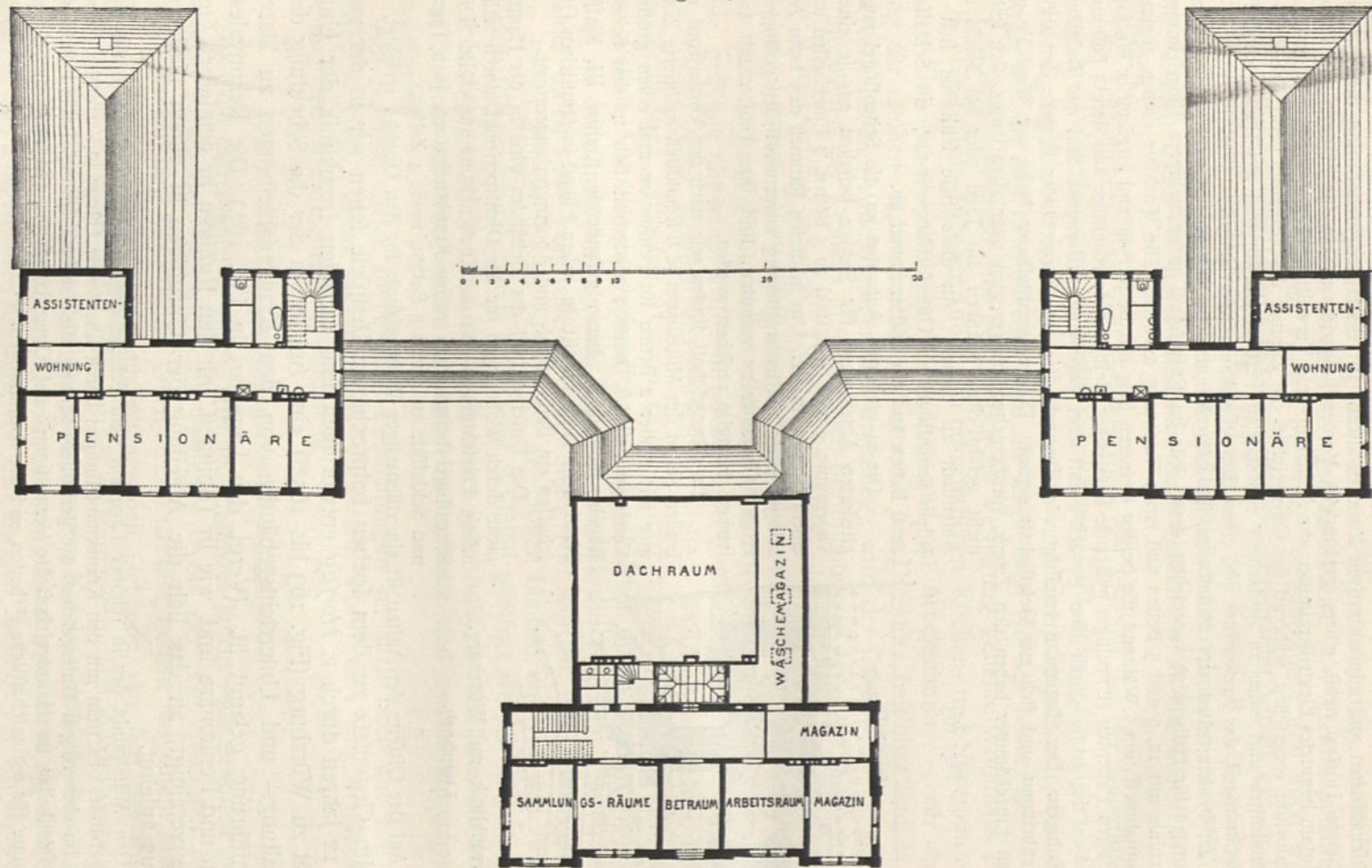
Obergeschoß.
