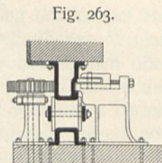
Gleitwerk von der Univeritäts-Sternwarte zu Bonn.
