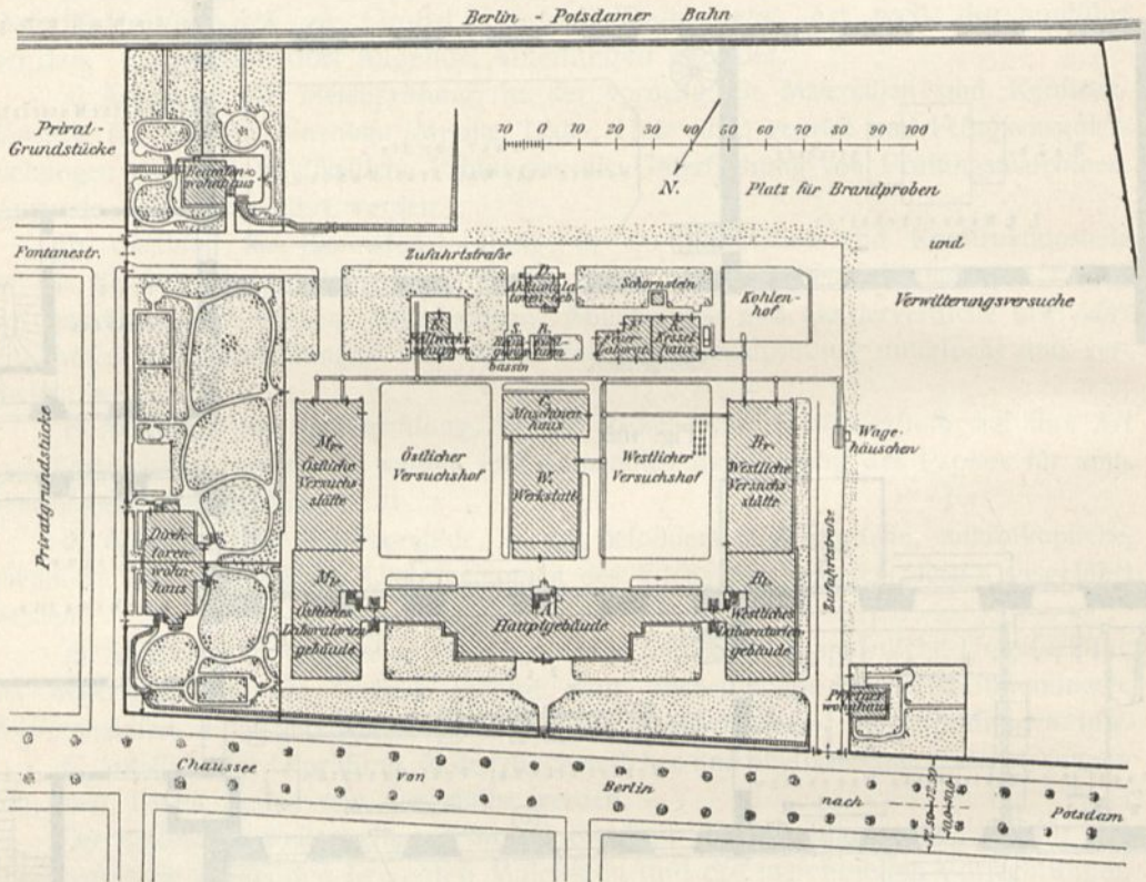
Königliches Materialprüfungsamt der Technischen Hochschule Berlin zu Groß-Lichterfelde-West 98) . Lageplan. Arch.: Guth.
