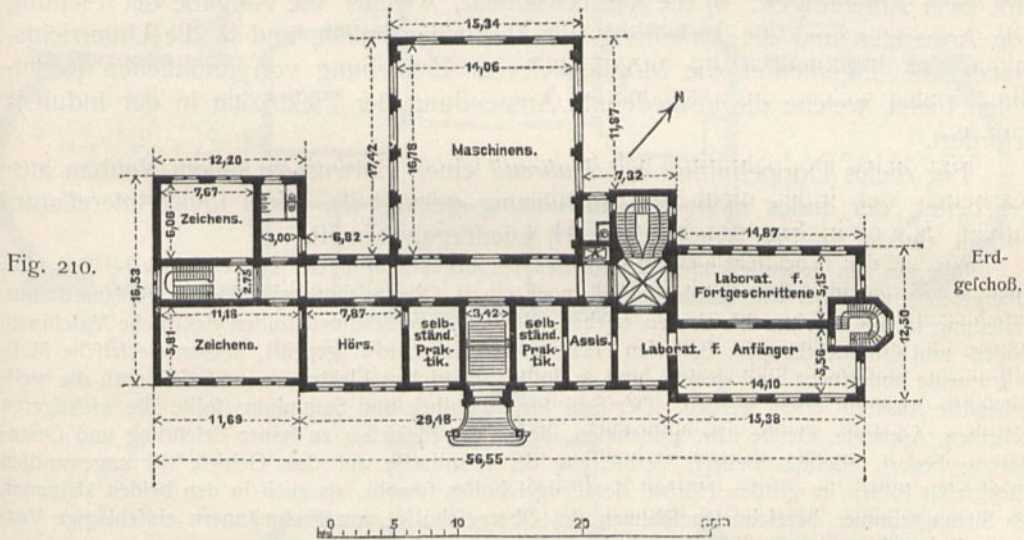
Elektrotechnisches Institut der Technischen Hochschule zu Danzig 154 ).
