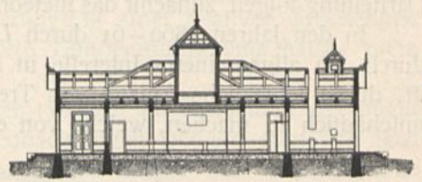
Längenschnitt.
