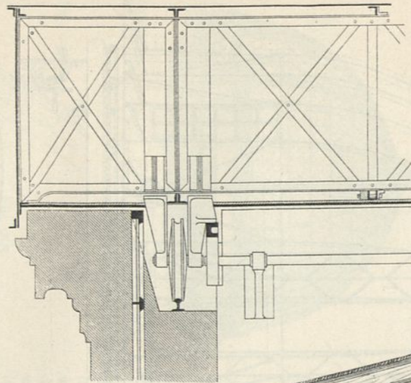
Gleitvorrichtung des Schiebedaches über dem Meridianfaal des afro-phyikalischen Observatoriums zu Bordeaux (Fig. 333 u. 334).
