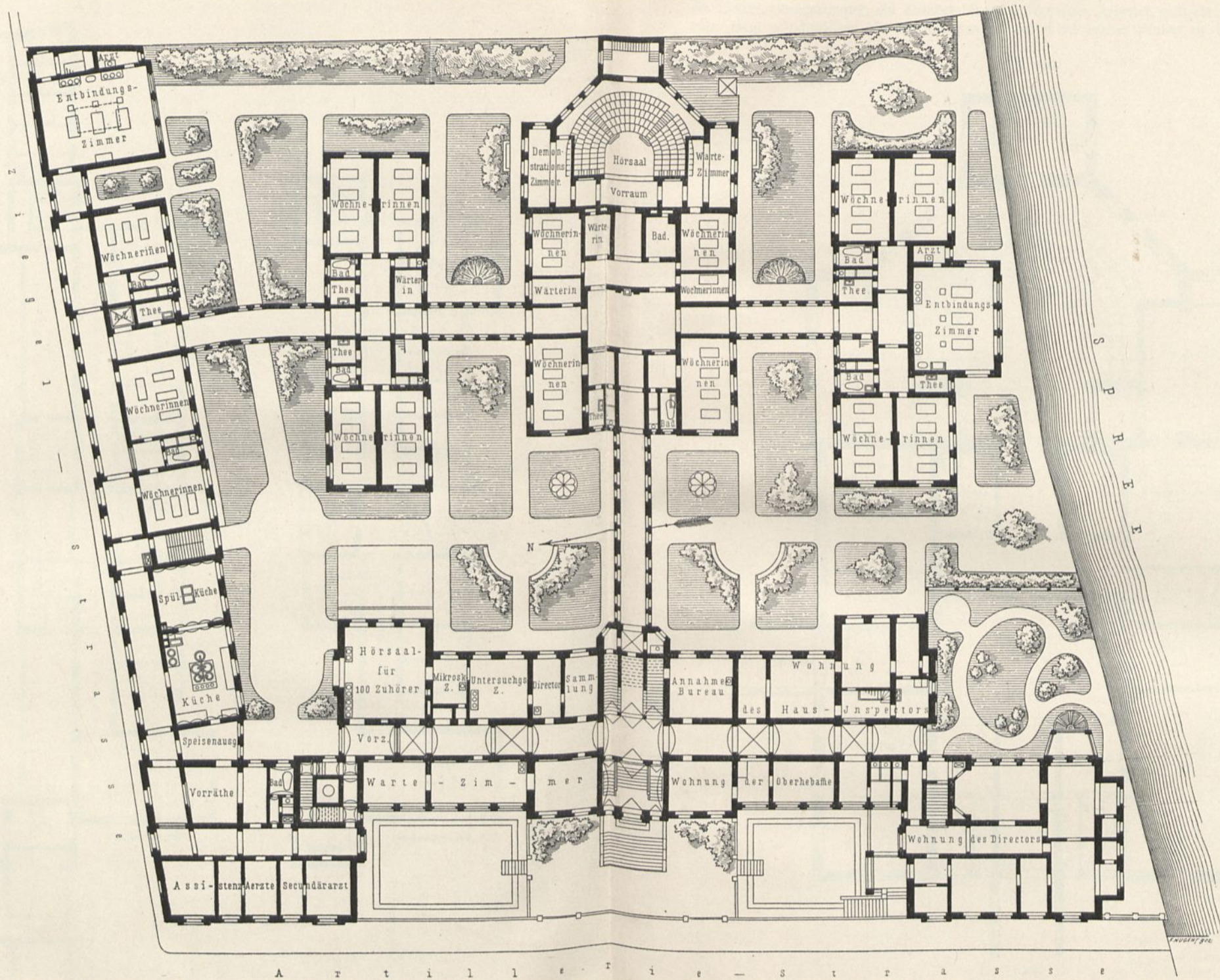
Erdgeschoß.
