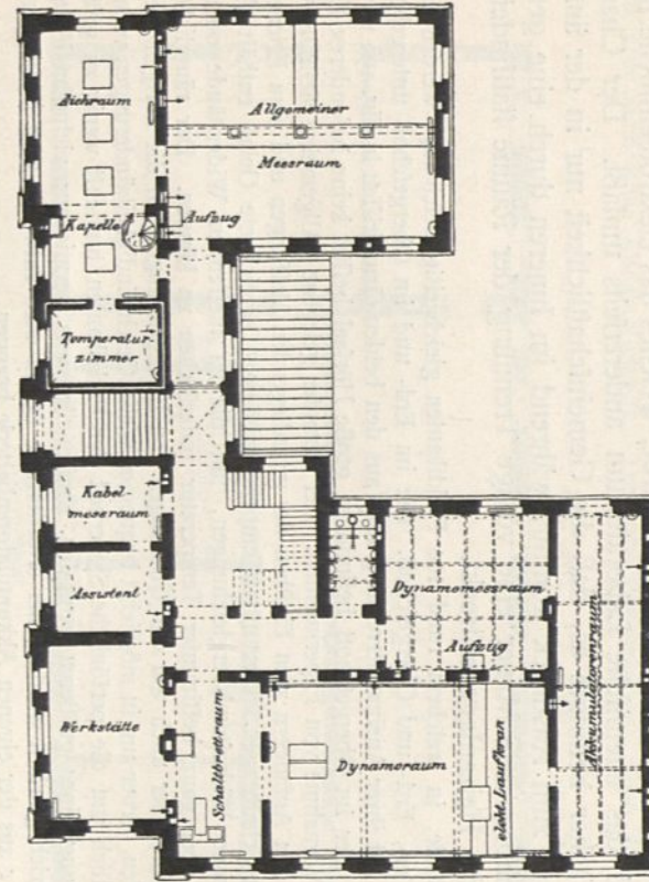
Obergeschoß.
