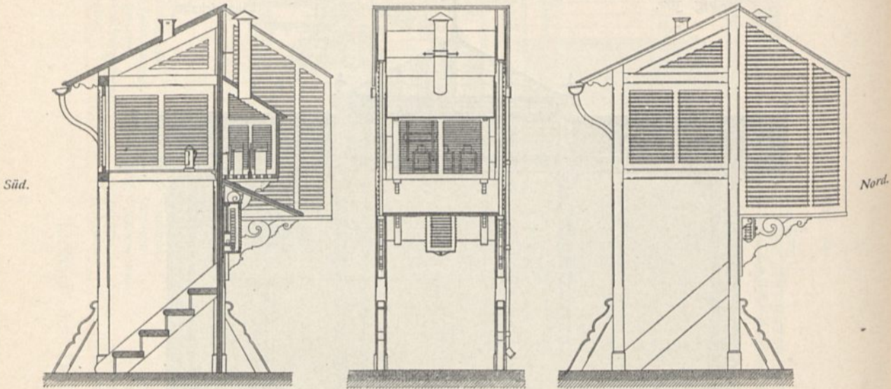
Thermometerhütten auf dem Wafferbecken der Deutschen Seewarte bei Hamburg 247) .
