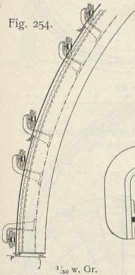
Dachrippe Führungsrolle für die Schiebeläden an der großen Drehkuppel des Observatoriums zu Bordeaux.
