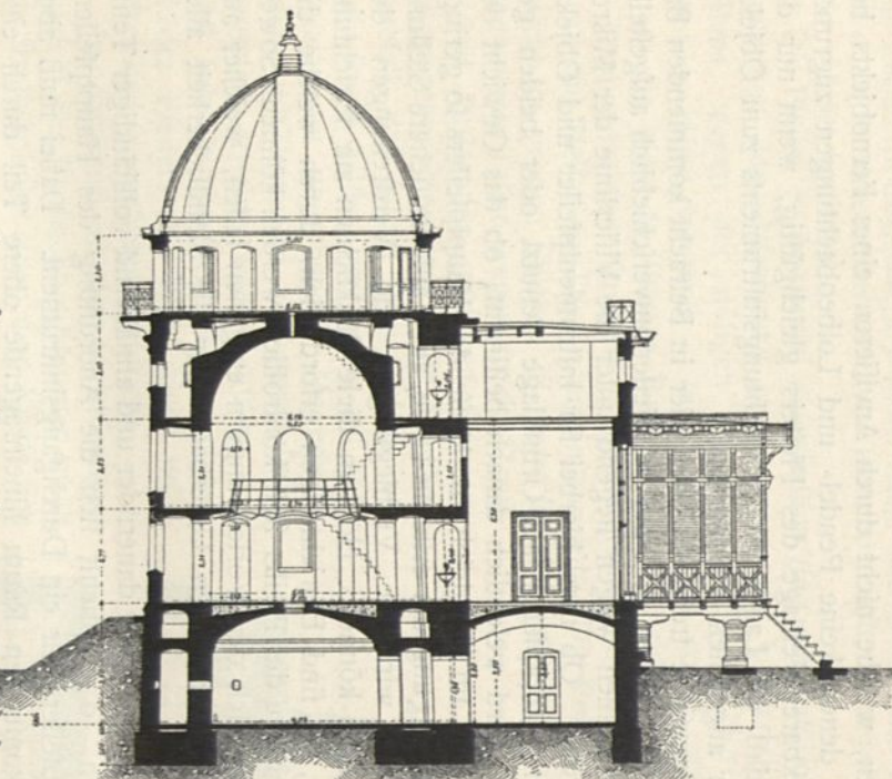
Östlicher Turm.
