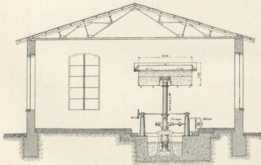
Schnitt A-B.
