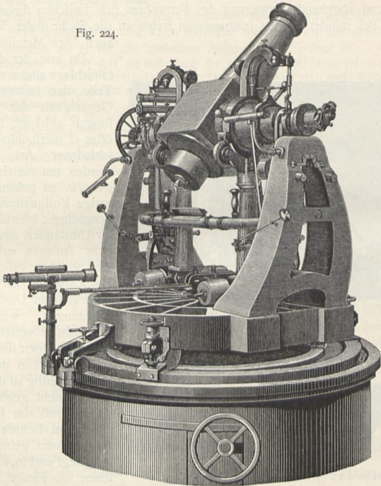
Universaltransit von Carl Bamberg in Berlin 109) .
