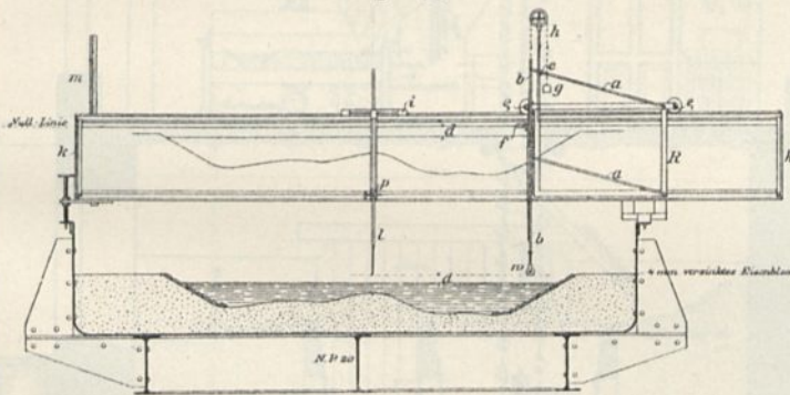
Veruchserinne mit der Vorrichtung zum Aufzeichnen der Querprofile 135) .
