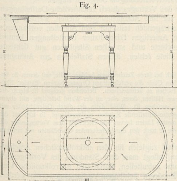
Leichtentisch im anatomischen Hörsaal zu Straßburg 6) . 1/25 w. Gr.
