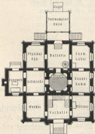
Erdgechoß.
