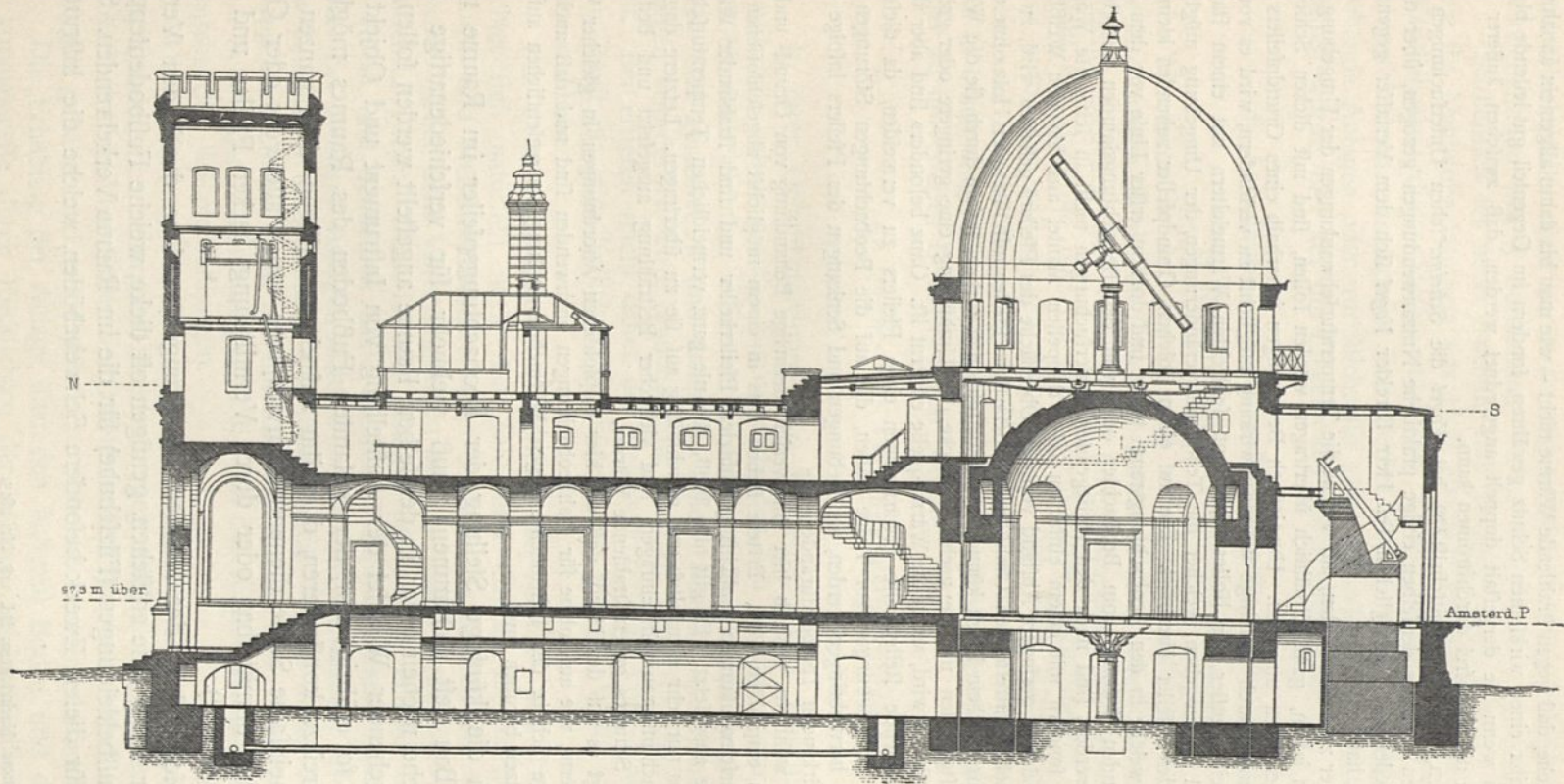
Meridional-Schnitt 178) .
