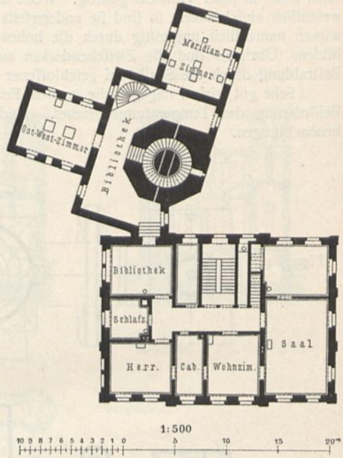
I. Obergeschoß.
