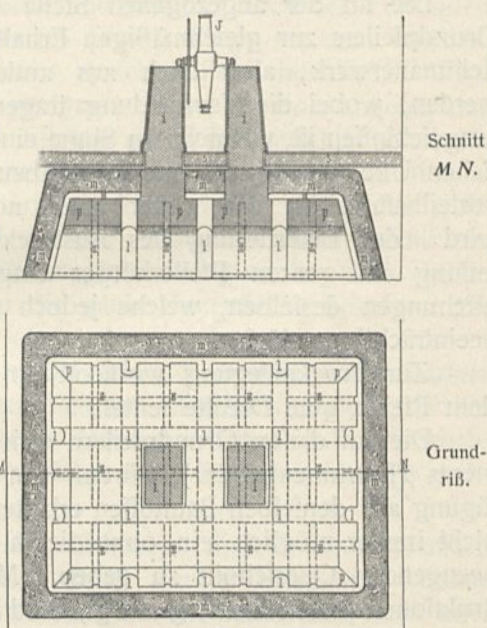
Grundpfeiler für ein Durchgangsinstrument.
