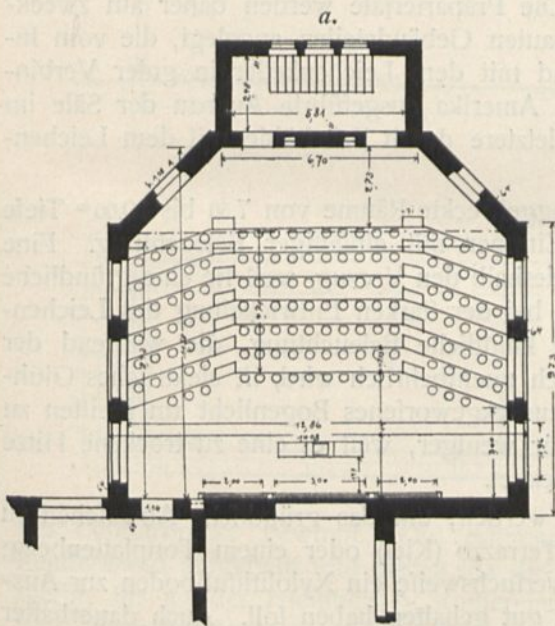
Hörfaal.
