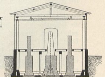
Querschnitt.
