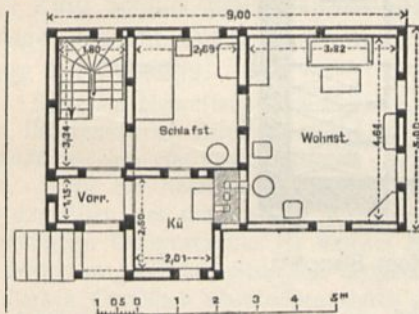
I. Obergeschoß.
