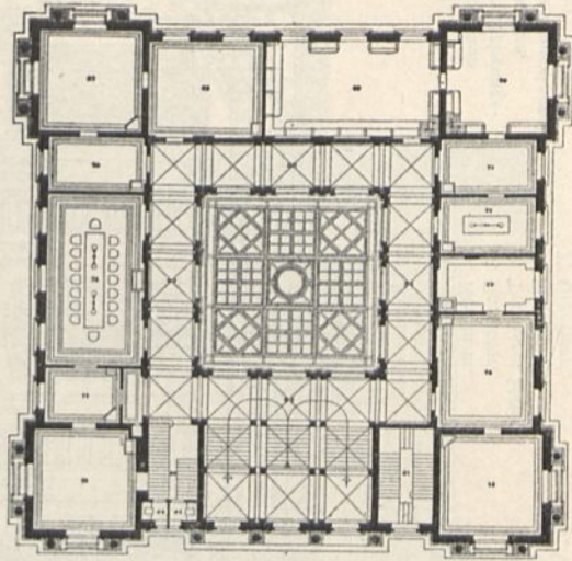
I. Obergechoß
