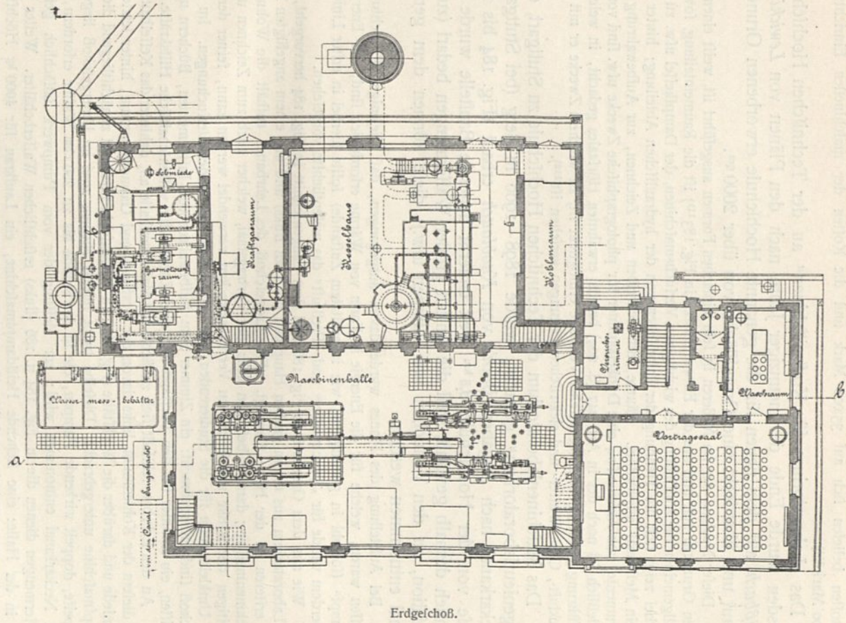
Ingenieurlaboratorium an der Technischen Hochschule zu Stuttgart 113) .
