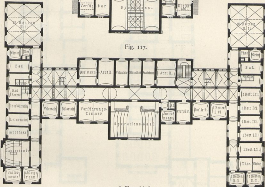
I. Obergeschoß.
