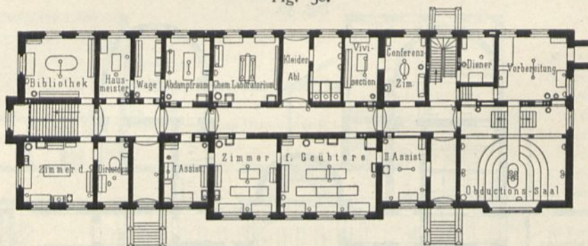
Erdgeschoß.
