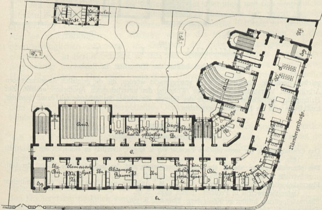
Erdgeschoß.
