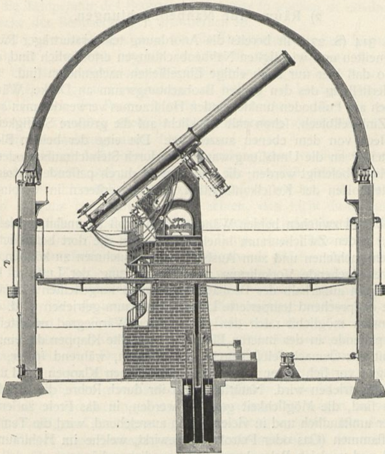
Drehkuppel des Lick -Observatoriums in Kalifornien 186 ).
