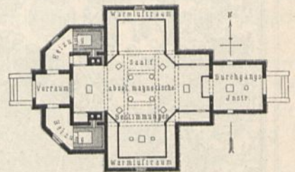
Grundriß.
