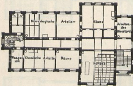
Hygienisches Institut der Universität zu Heidelberg 50) .
