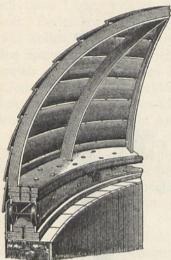
Gleitwerk vom Warner's Observatorium zu Rochester 197) .
