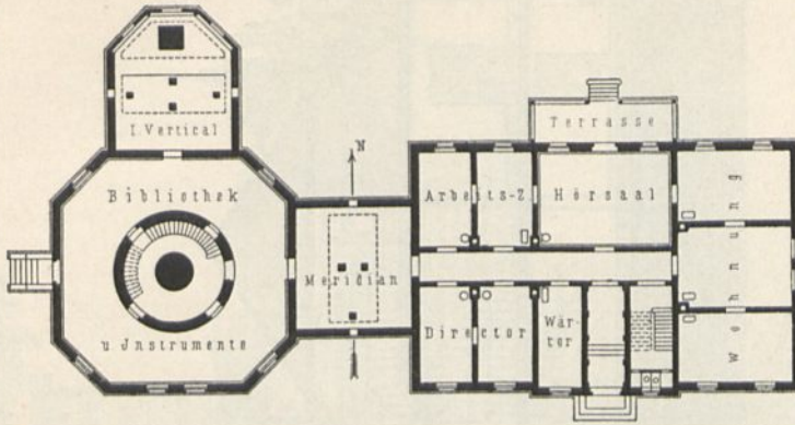
Univerfitäts-Sternwarte zu Leipzig.
