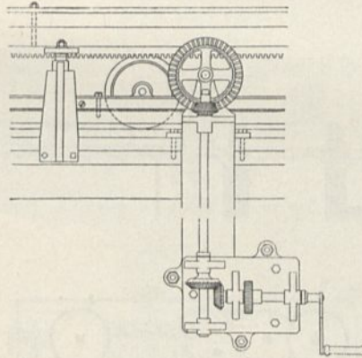
Gleit- und Triebwerk.
