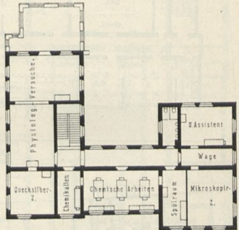
Obergefchoß.
