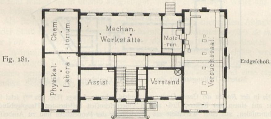
Eidgenössische Anstalt zur Prüfung von Baumaterialien zu Zürich 100 ).
