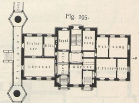
Hauptgebäude. — Erdgeschoß.
