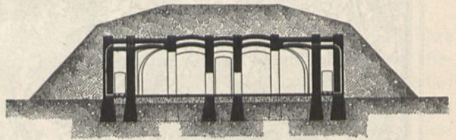
Längenschnitt.
