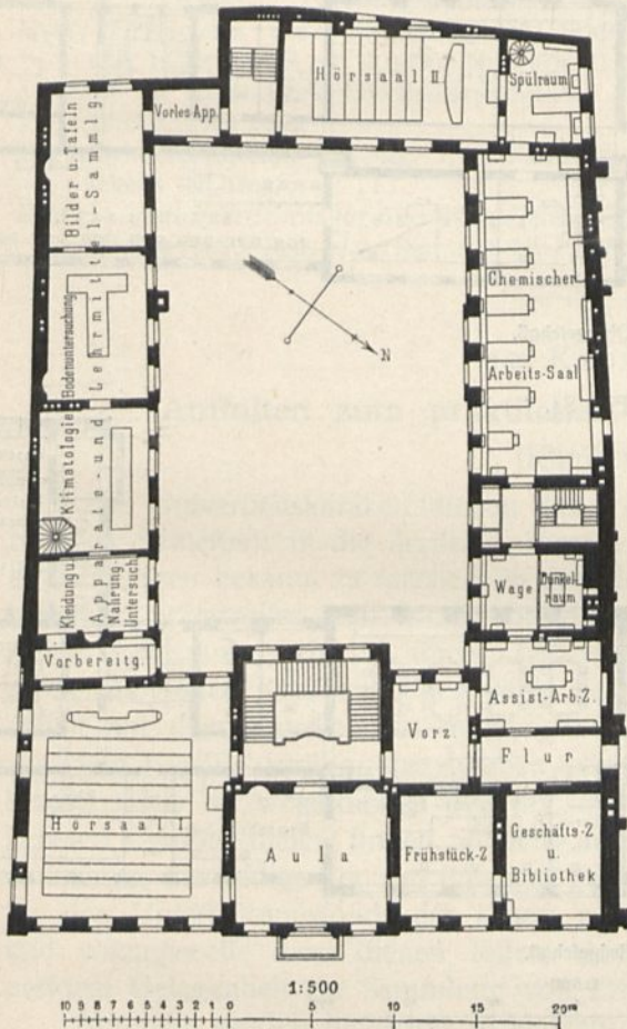
Hygienisches Institut der Universität zu Berlin 52 ).
