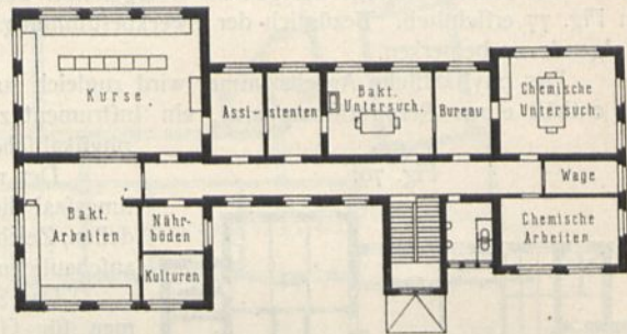
Obergeschoß.
