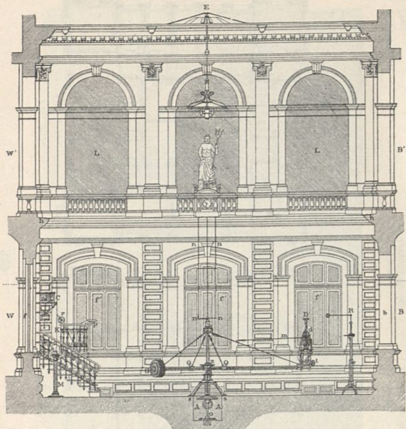
Längenschnitt.
