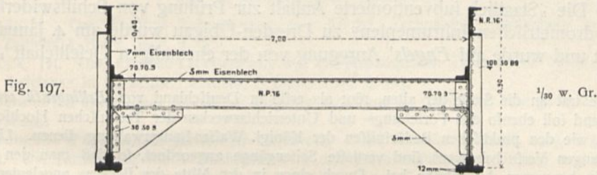
Querchnitt durch das Versuchsgerinne 139) .
