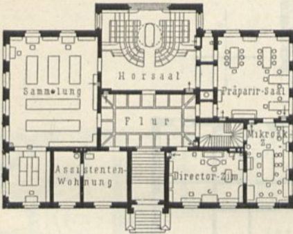
Anatomiegebäude der Universität zu Kiel.
