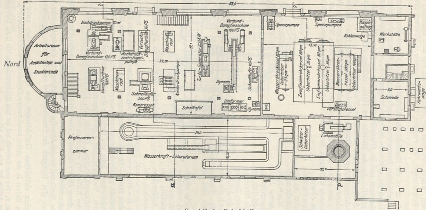
Grundriß des Erdgeschosses.
