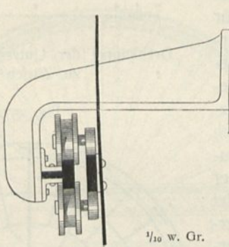
Dachrippe Führungsrolle für die Schiebeläden an der großen Drehkuppel des Observatoriums zu Bordeaux.
