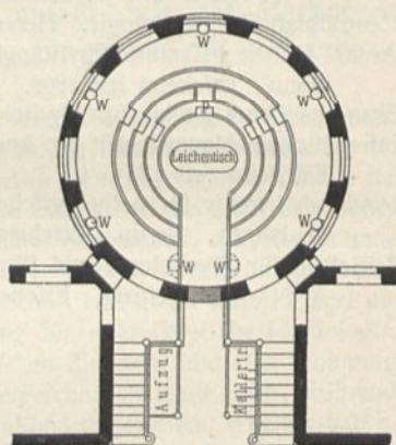
Pathologischer Obduktionsaal.
