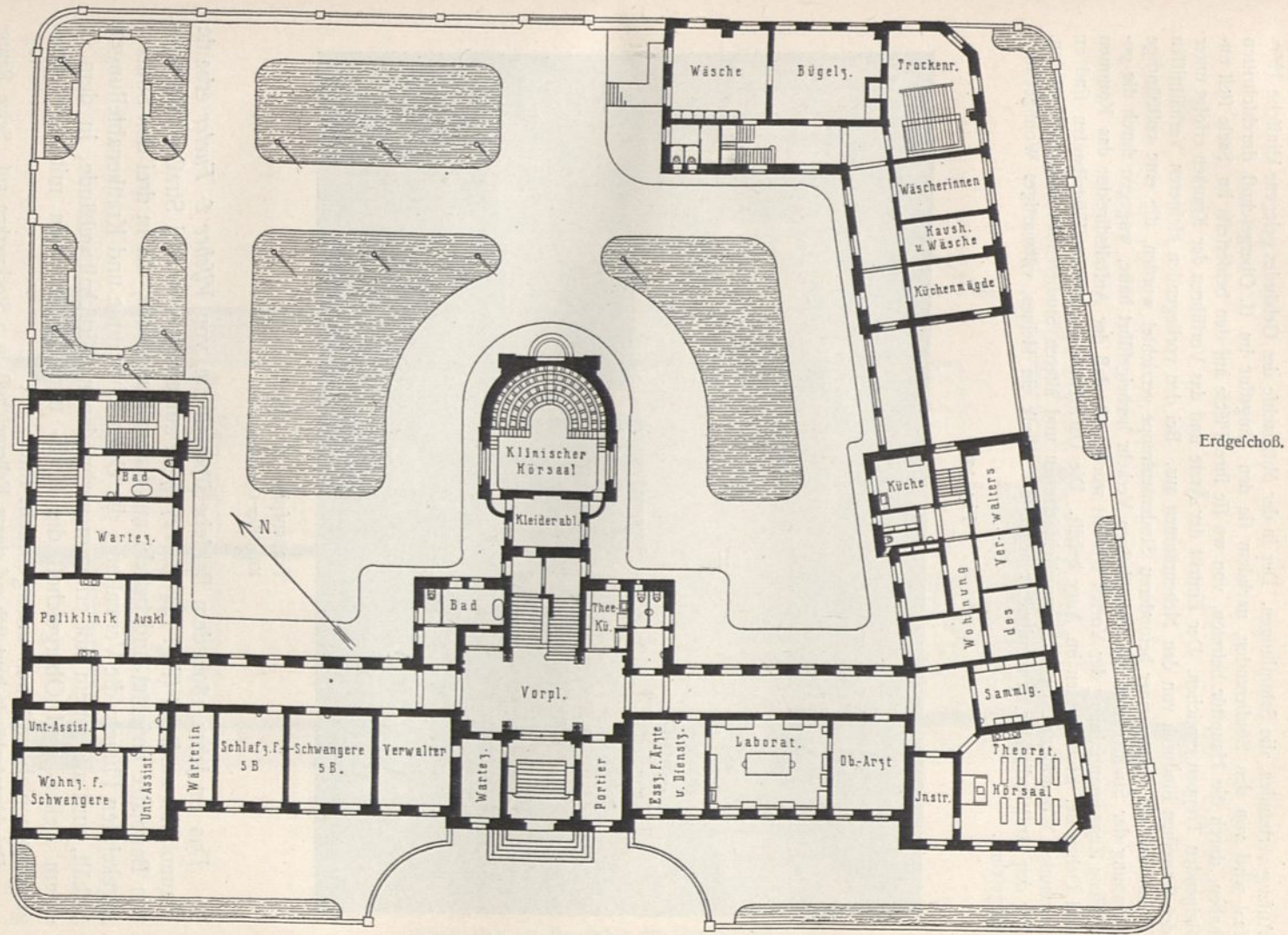
Frauenhospital zu Basel 71).
