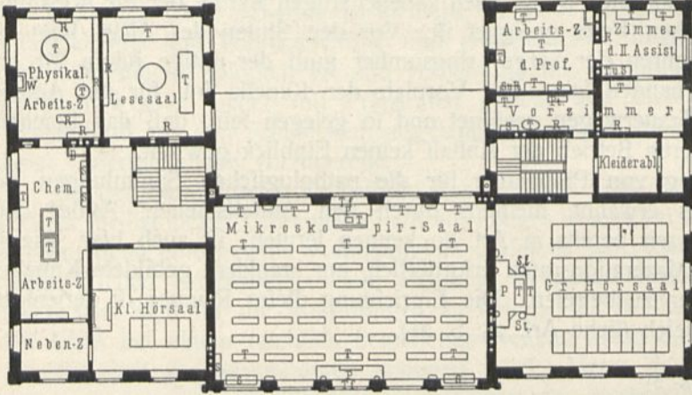
Obergechoß.
