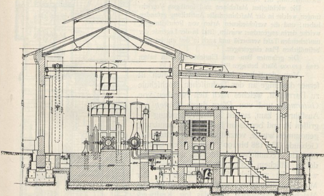
Maschinenlaboratorium der Technischen Hochschule zu Berlin.
