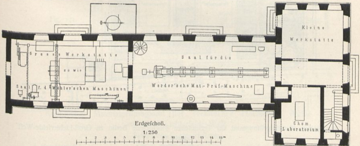
Mechanisch-technisches Laboratorium der Technischen Hochschule zu München.
