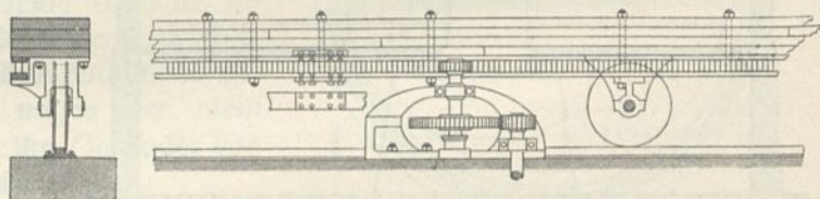
Gleit- und Triebwerk von der Sternwarte zu Zürich 195 ).
