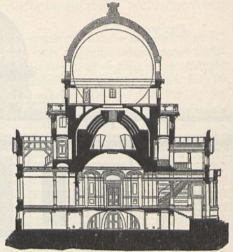
Querschnitt.
