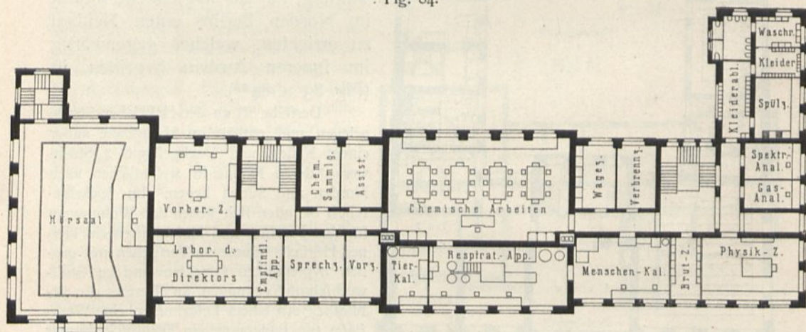
Erdgehoß.
