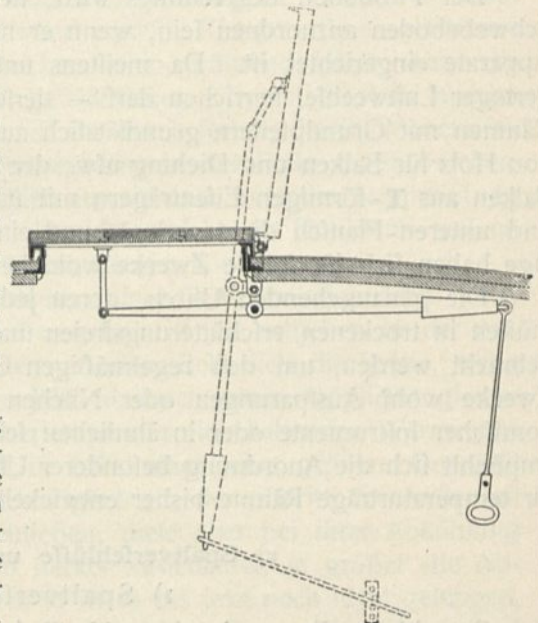
Dachklappe vom astronomischen Observatorium der Technischen Hochschule zu Wien 186) .
