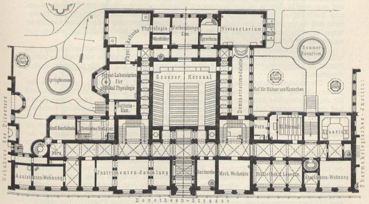
Erdgechoß.
