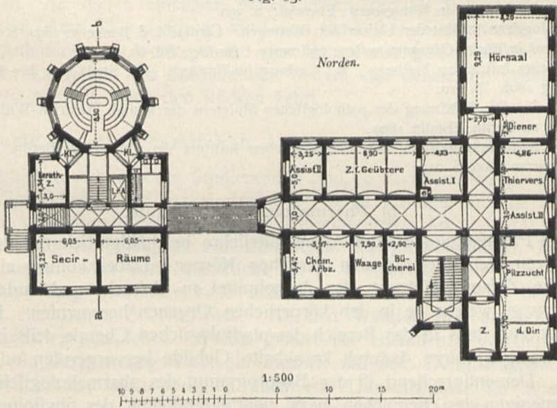
Erdgechoß.
