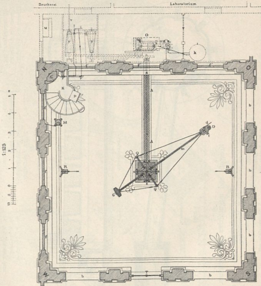
Grundriß.
