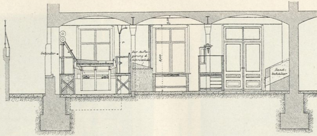
Querschnitt nach E F.
