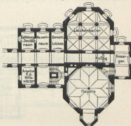
Obduktionshaus. Untergeschoß.
