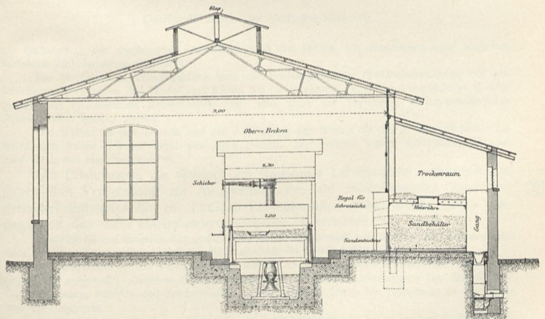
Schnitt C-D.
