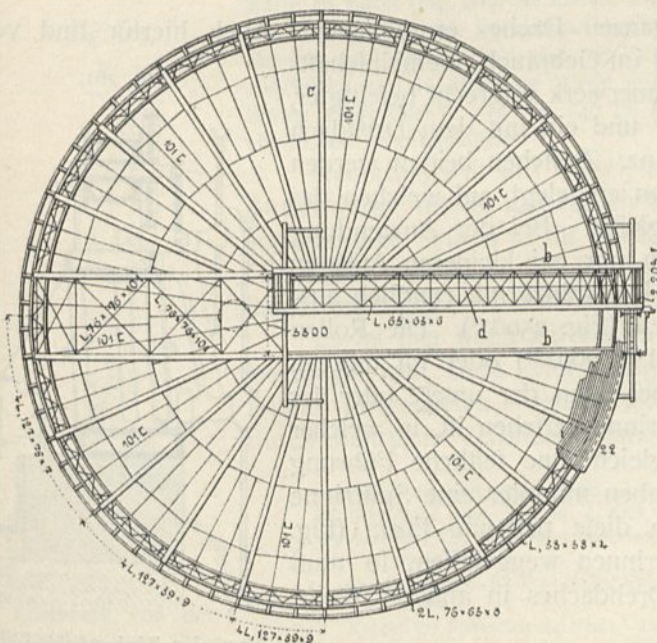
Große Drehkuppel des Observatoriums zu Lake Geneva 193) .
