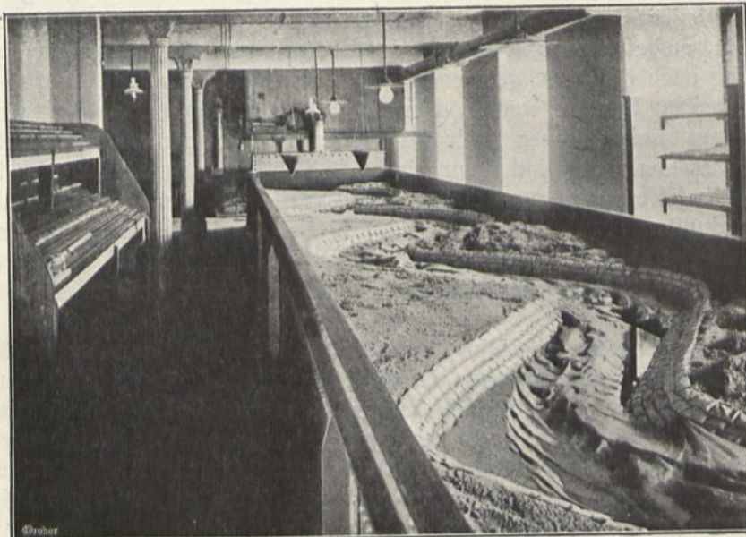
Blick in das Versuchserinne nach Beendigung eines Modellverfuches. (Stromaufwärts.)
