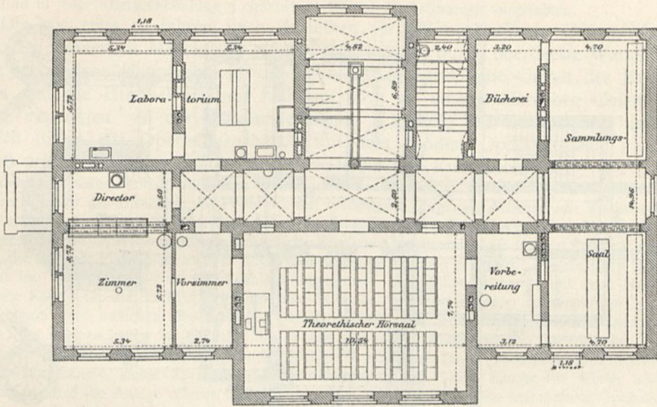
Obergeschoß.
