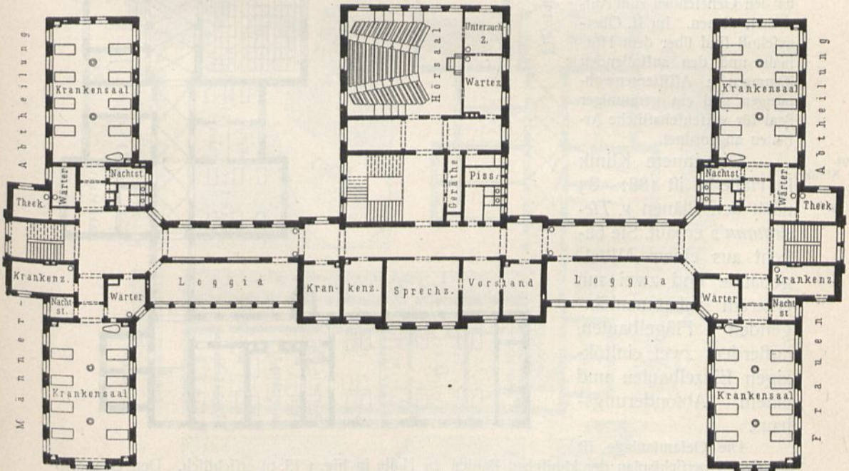
I. Obergeschoß.
