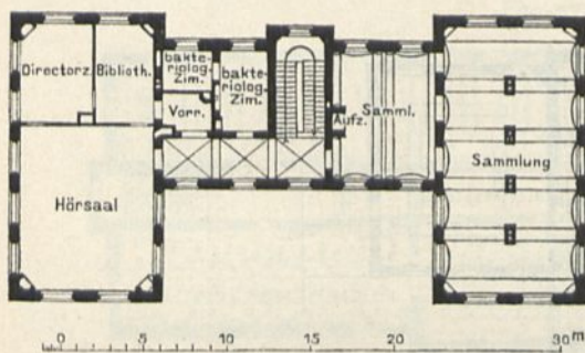
Lehrgebäude. II. Obergeschoß.
