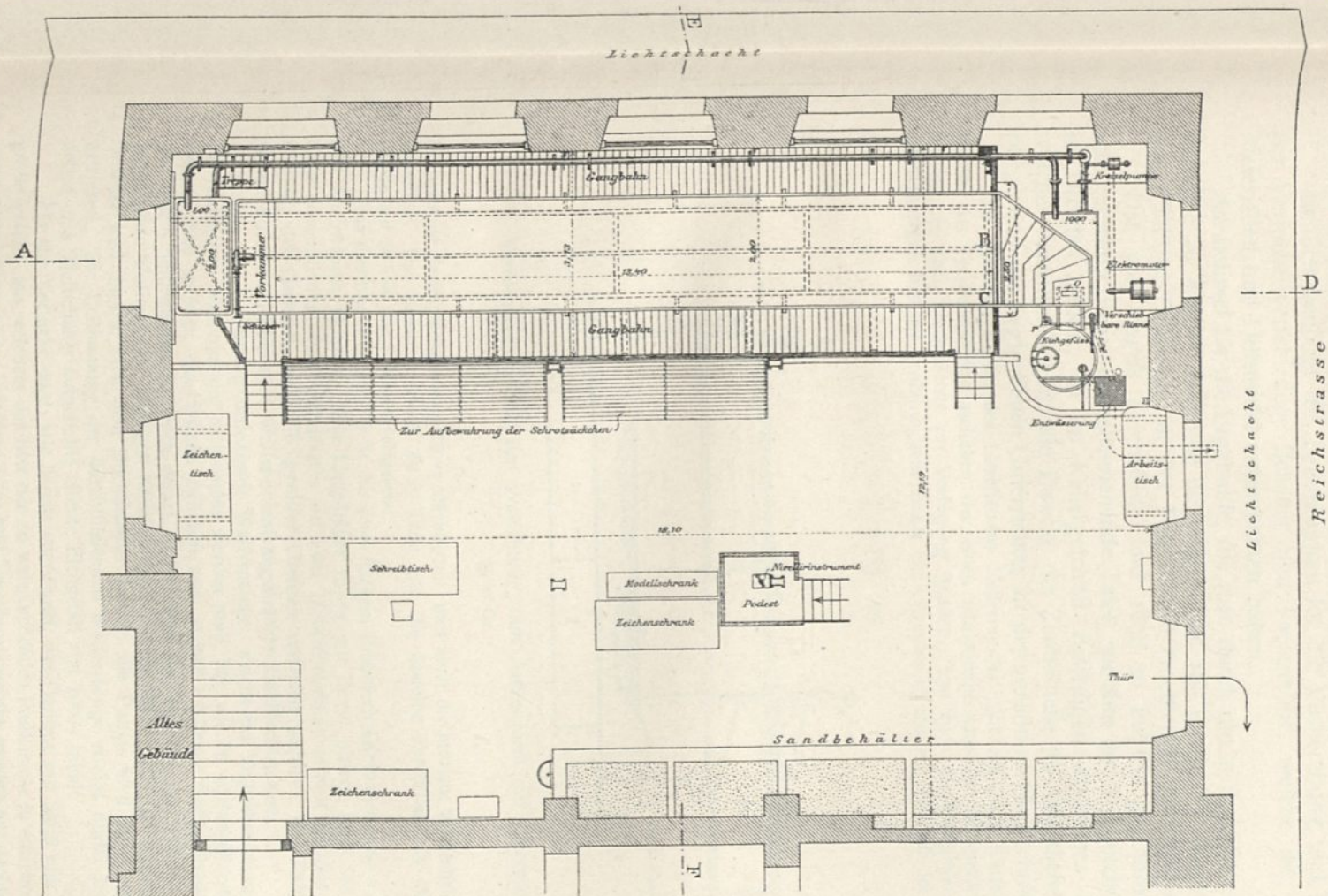
Grundriß.
