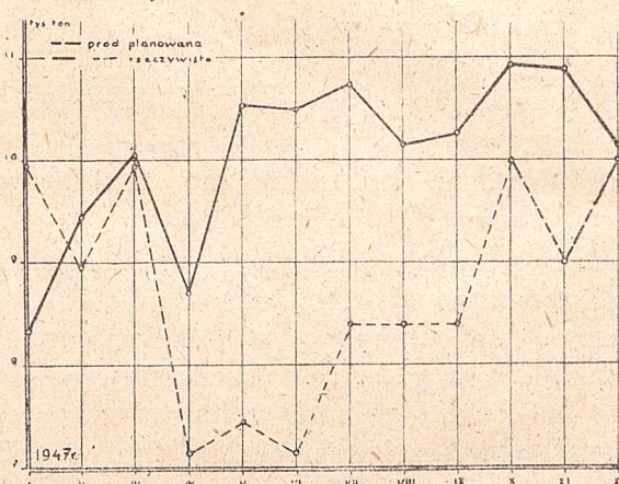
Produkcja azotniaku
