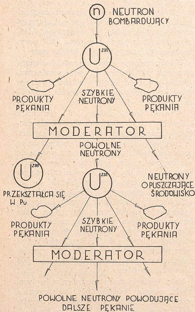
Schemat reakcji łańcuchowej w stosie uranowo-grafitowym w-g H. D. Smytha: Atomic Energy for Military Purposes.
