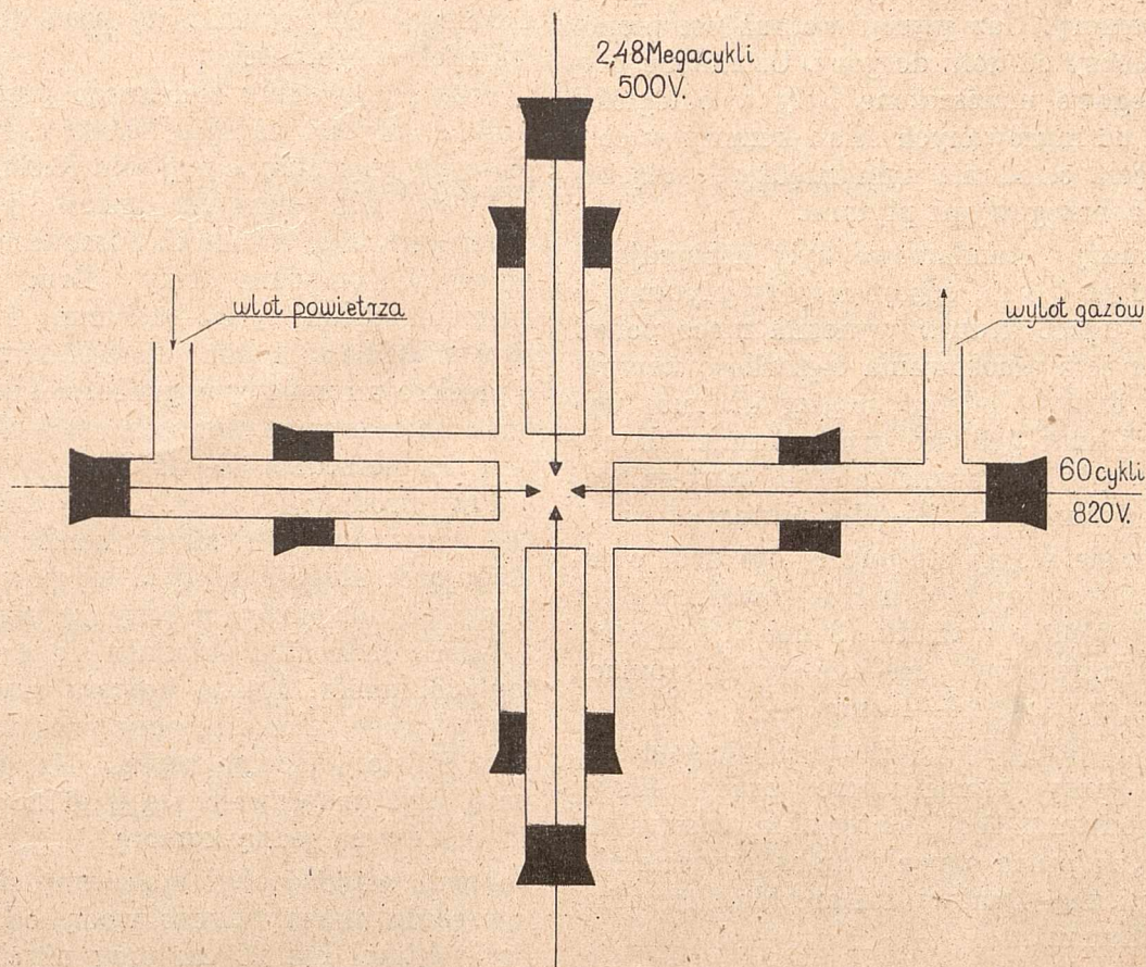
Schemat aparatury laboratoryjnej.
