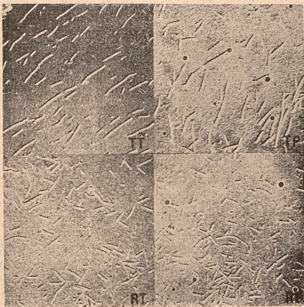
Wirus mozaiki tytoniowej. Stanley and Anderson: Electron microscopy of viruses.
