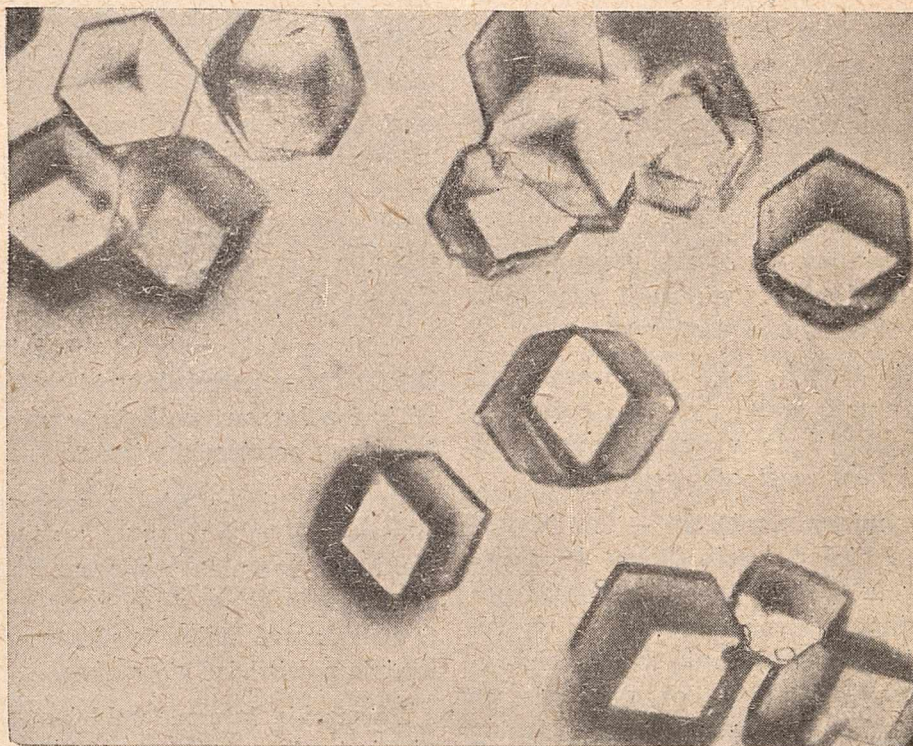
Krystały wirusa kędzierzawki ziemniaczanej (224-krotne powiększenie zdjęcia mikroskopu elektronowego). Stanley, Chem. Eng. News, 25 (1947).
