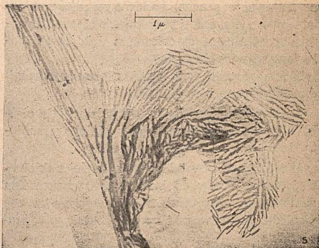
Zlepione pałeczki wirusa mozaiki tytoniowej. Stanley and Anderson: Electron microscopy of viruses.
