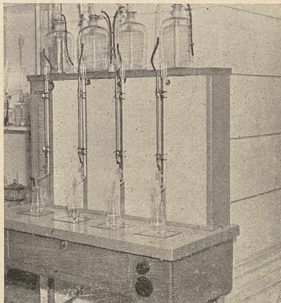
Stół do miareczkowania z mieszadłem magnetycznym NRD
