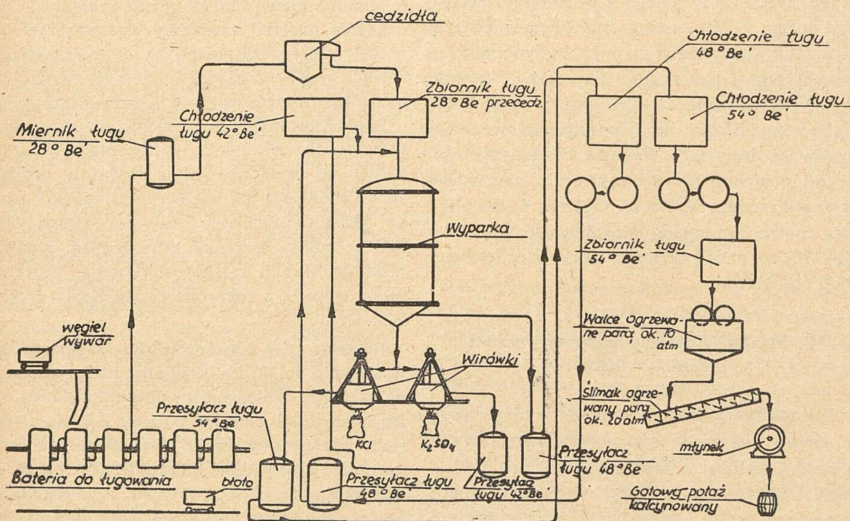
Schemat rafinerii soli potasowych
