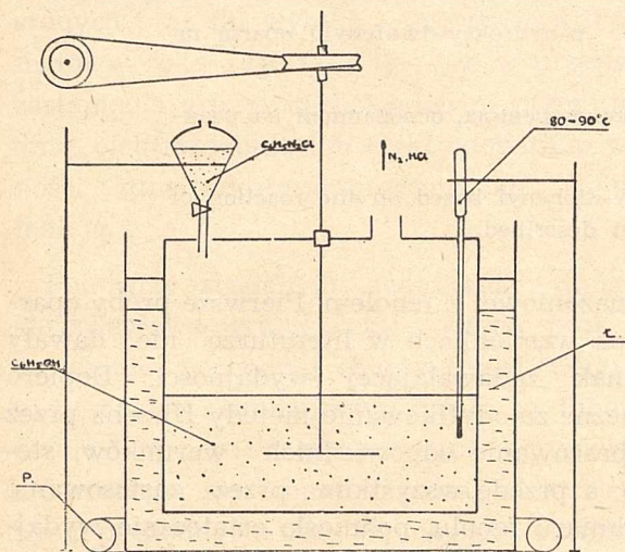
Rys. 2. Reakcja soli dwuazoniowej z fenolem Ł — łaźnia wodna; P — palnik gazowy
