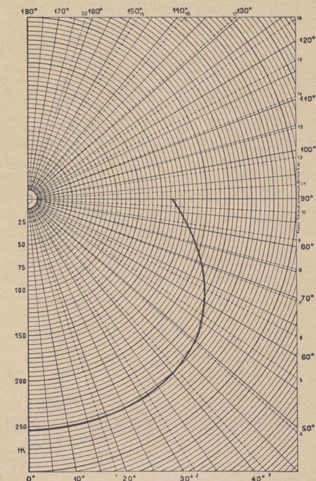
Rys. 2. Siatka do obliczania strumienia świetlnego (Franz Schmidt & Haensch, Berlin) z wrysowaną krzywą światłości 3-płom. palnika wiszącego wbudowanego.
