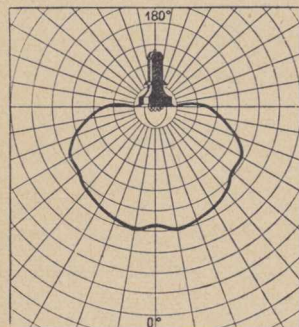
Lampa wisząca z palni- kiem grupowym.
