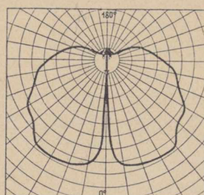
Palnik wiszący wbudowany.
