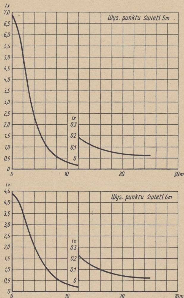
Rys. 10. Krzywe jasności poziomej przy nowoczesnych lampach gazowych, w przeliczeniu na 100 HK \square , w odstępach 0 do 30 m od stopy lampy, wysokość punktu świetlnego 5 do 9 m.
