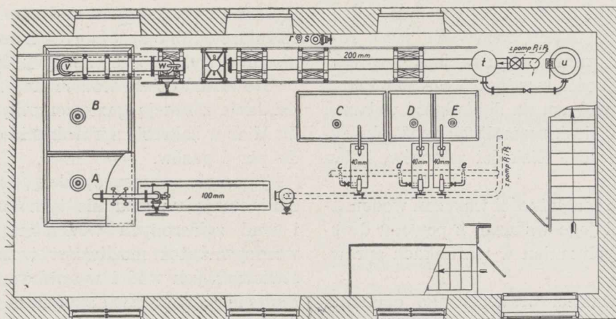
Rys. 2. Plan laboratorium wodomierzowego GUM.
