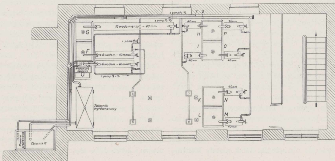
Rys. 3. Plan laboratorium wodomierzowego GUM.
