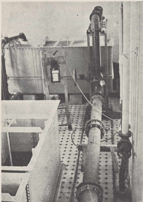
Rys. 6. Sprawdzanie wodomierza Venturi'ego.
