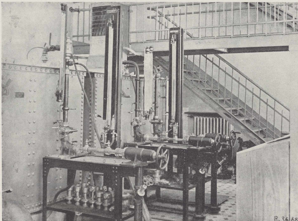
Rys. 4. Układy miernicze do wodomierzy 40 mm.
