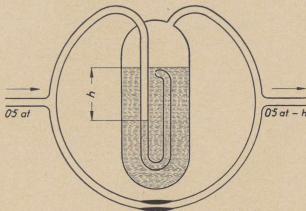
Rys. 2. Przyrząd dozujący chlor.
