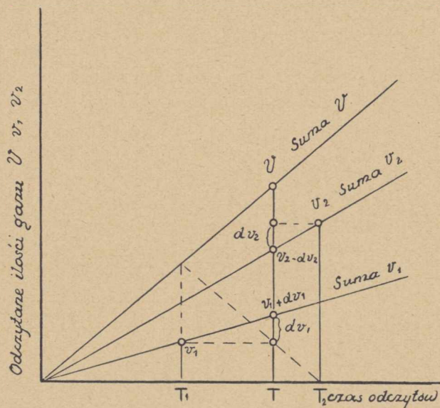
Rys. 2. Zależność między czasem odczytywania gazomierzy a ilością odczytanego gazu.
