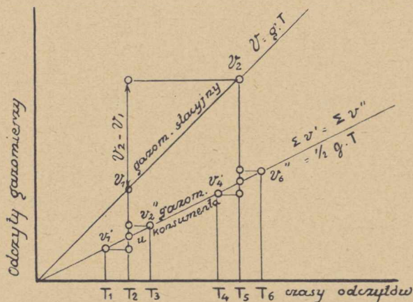
Rys. 3. Zależność między czasami odczytów miesięcznych a ilością odczytanego gazu.
