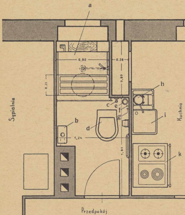
Rys. 2. Rozplanowanie części gospodarczej małego mieszkania. a — wnęka do mycia i natrysku, b — wiszący piecyk gazowy, c — spłuczka, d — klozet, e — przewód kanalizacyjny, f — przewód wodociągowy, g — przewód gazowy, h — mały automatyczny grzejnik wody gazowy, i — zmywak i zlew, k — kombinowy piec kuchenno-gazowy.
