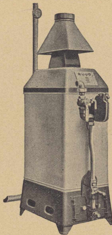
Rys. 22. Kocioł Ruuda.
