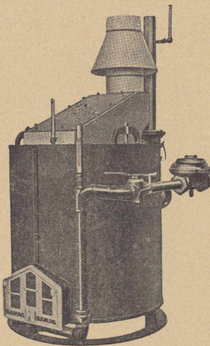
Rys. 23. Kocioł Bamaga.
