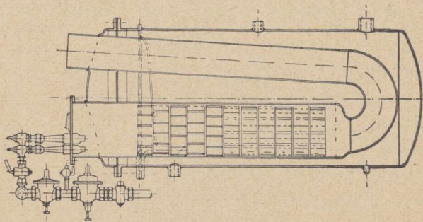
Rys. 26. Przekrój boileru typu „Gasstrahl“.
