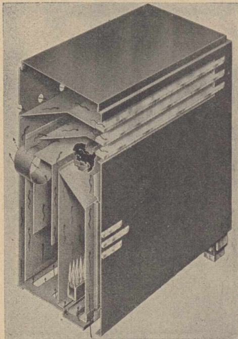
Rys. 17. Piec cyrkulacyjno-powietrzny.
