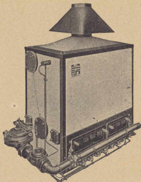
Rys. 21. Kocioł typu „Ideal”.
