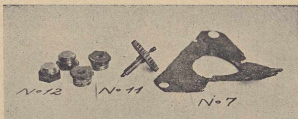
Rys. 3. Płytki potoczne, kółko zębate i gniazdko prowadzące oś skrzydełka, zniszczone przez korozję.
