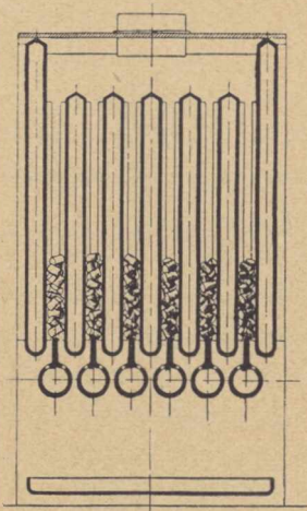
Rys. 20. Przekrój kotła „Phi”.
