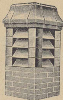
Rys. 29. Nasada kominowa.
