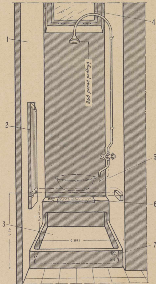
Rys. 1. Wnęka do mycia i natrysku. 1 — wyprawa cementowa, do wysokości okna malowanie olejne, 2 — ruszt drewniany, 3 — wanienska do natrysku i mycia nóg, 4 — wysoko umieszczone okno z dźwignią, 5 — bateria wodna z rurą ruchomą, zakończoną nasadką dla węża, 6 — wkładka drewniana, służąca jako ławeczka, 7 — wypust z rurką przelewową.
