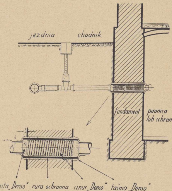
Rys. 1. Typowe gazo- i wodoszczelne przejście rurociągu przez mur fundamentowy.
