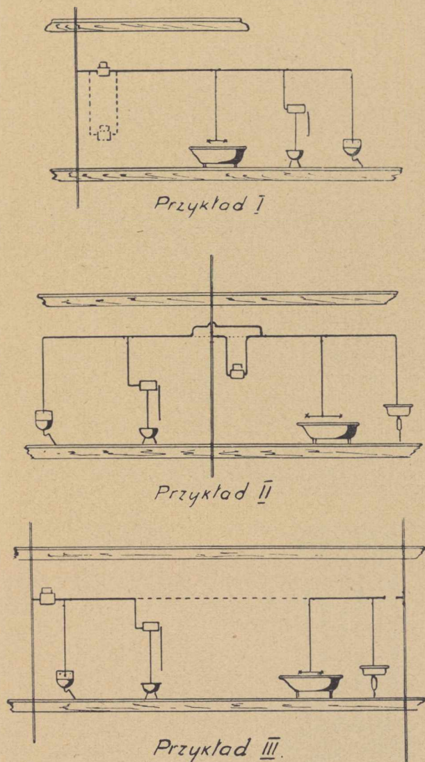
Rys. 6. Typowe rozwiązania ustawienia odliczników.
