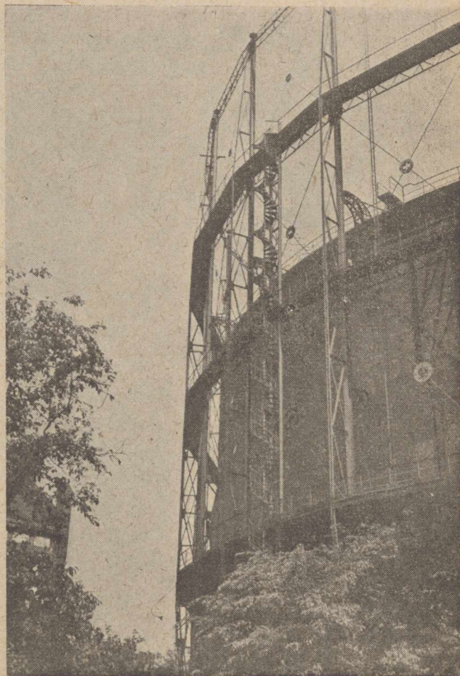
Rys. 6. Zbiornik poj. 110.000 m.
