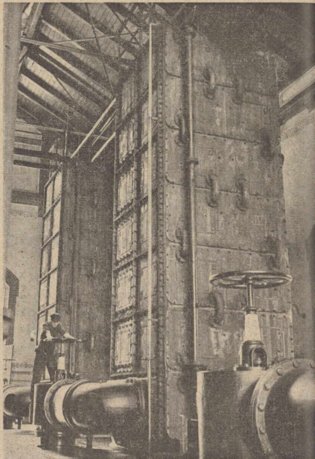
Rys. 4. Chłodnice wodne.
