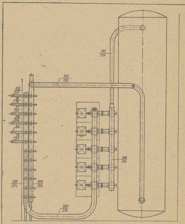
Rys. 2 — dół
