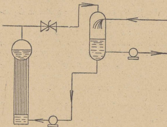
Rys. 8. Schemat grzania wody obiegowej w kaskadowym wymienniku ciepła
