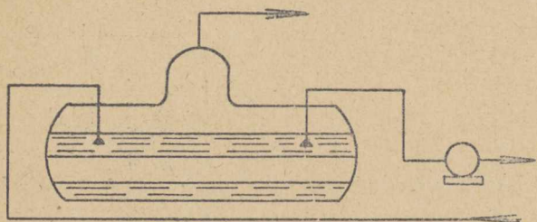
Rys. 7. Schemat pobierania pary z kotła pracującego na ogrzewanie
