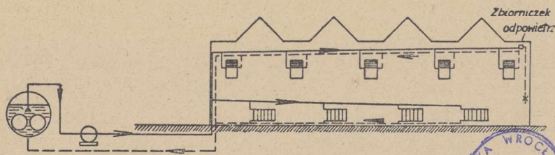
Rys. 5 Schemat ogrzewania hali wagonowej
