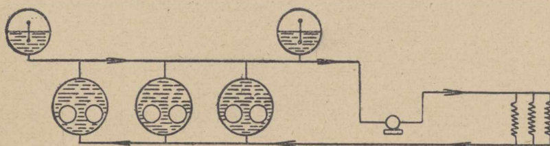
Rys. 2. Schemat połączeń kotłów ze zbiornikami wodno-powietrznymi
