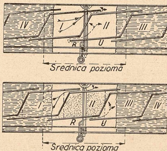
Rys. 3. Rozwinięcie przekroju przez komory bębna mierniczego I, II, III, IV — komory, U — przedsionek, R — rurka wlotowa.
