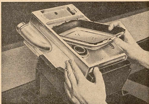
Rys. 5. Komora miernicza.
