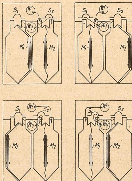
Napętnienie i opróżnienie gazomierza suchego typu Elsler. Wl — wlot; Wy — wylot; M 1 , M 2 — membrany; S 1 , S 2 — suwaki.
