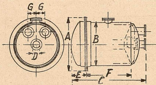
Rys. 2. Gazomierz duży, mokry
