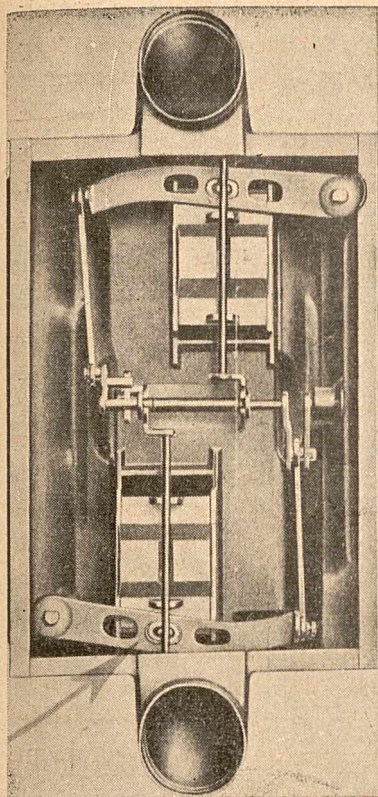
Rys. 6. Komora suwakowa
