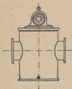
Rys. 16. Gazomierz „Rotary”
