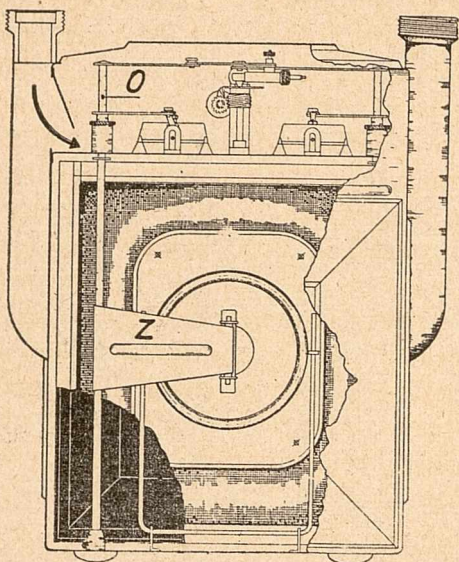
Rys. 4. Gazomierz suchy membranowy (miechowy) Fabryki Toruń
