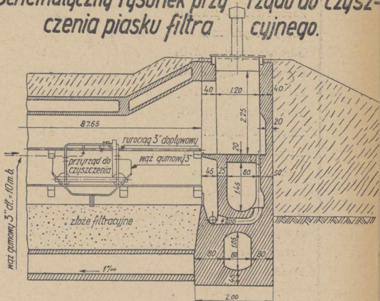
Przekrój podłużny filtra przy komorze dopływowej.
