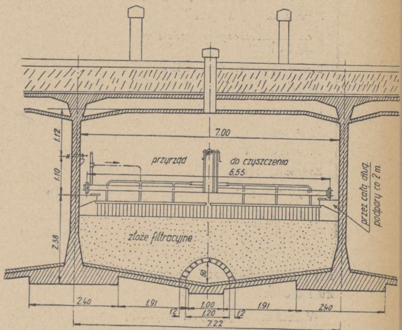
Przekrój poprzeczny filtra.
