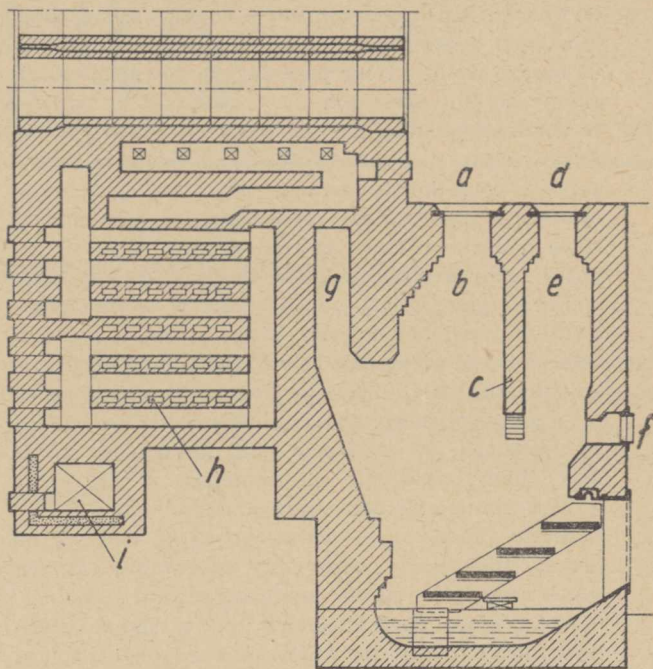
Rys. 1. — Przekrój generatora dla drobnych gat. koksu. a — otwór wsypowy dla koksu grubego, b — warstwa koksu grubego, c — ściana przedziałowa, d — otwór wsypowy dla koksu drobnego, e — warstwa koksu drobnego, f — dopływ powietrza, g — wyjście gazu generatorowego, h — rekuperacja, i — kanał dymny.
