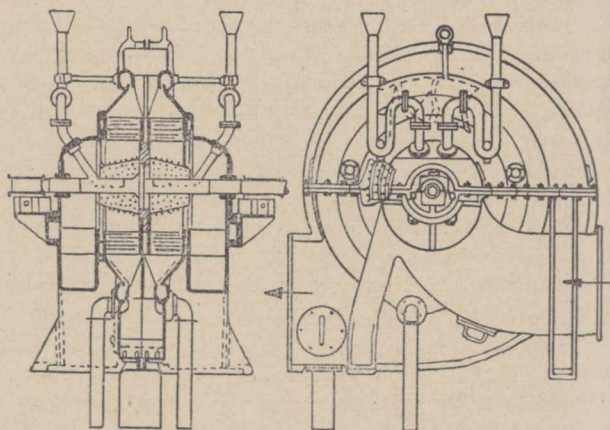
Płuczka Theisena.
