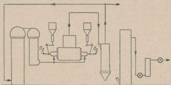
Rys. 2. Schemat procesu zgazowania pyłu węglowego systemem Koppersa.
