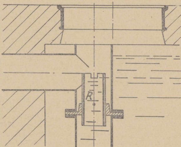
Przestawny przelew dołu rozdzielczego.
