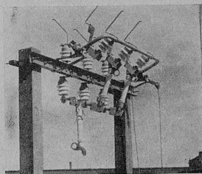
Wyłączniki i odłączniki słupowe, zwykłe i z bezpiecznikami
