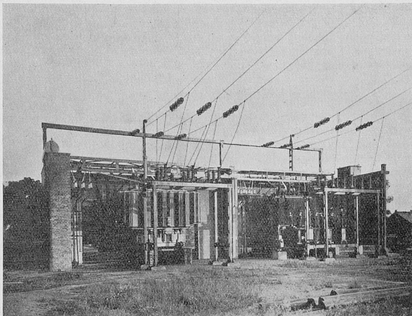
Rys. 6. Przetwórnica napowietrzna Katowice. Widok zewnętrzny.
