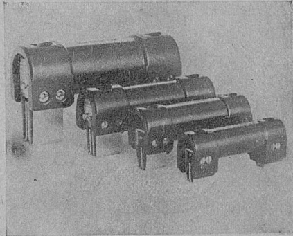
Bezpieczniki różnych typów prasowane z masy izolacyjnej
