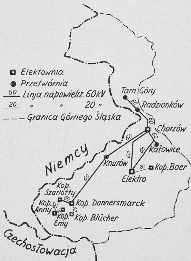
Rys. 1. Sieć 60 kV Górnego Śląska.
