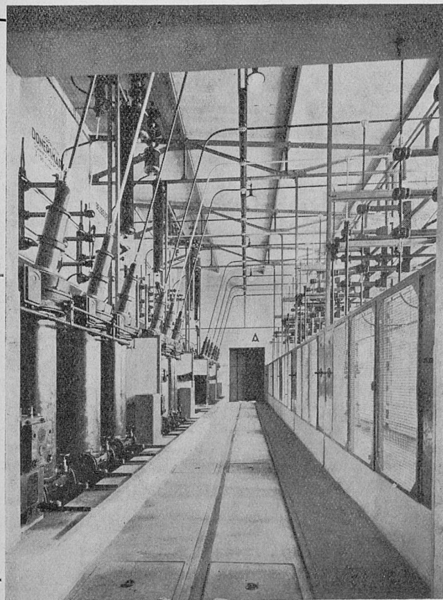
Rys. 5. Przekrój przez rozdzielnię przetwórnici Knurów.
