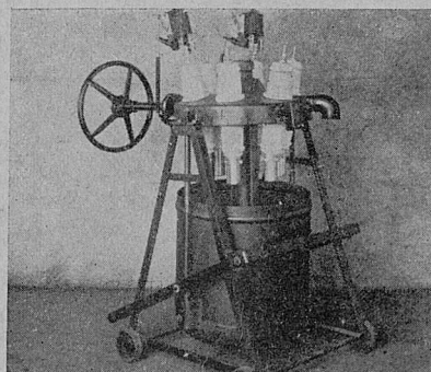
Wyłączniki olejowe dla napięć do 35 kV i mocy odłączalnej do 200 MVA
