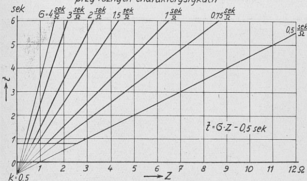
Rys. 8. Krzywe wartości ochronnych odgromników przepięciowych.
