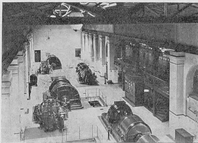
Rys. 2. Widok hali maszyn.
