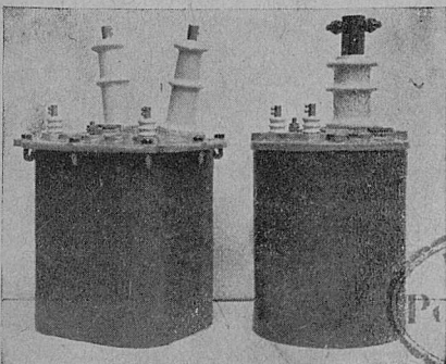
Transformatory miernicze prądowe do 6000 A i napięciowe do 35000 V
