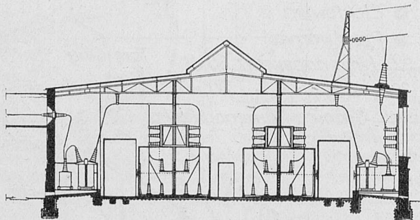
Rys. 2. Przekrój przez rozdzielnię przetwórnicy Chorzów.
