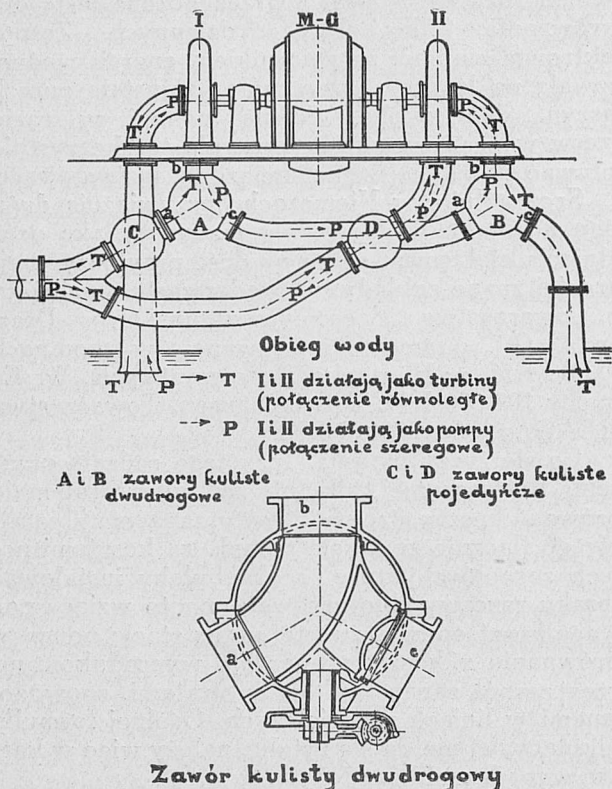
Rys. 1. Nowy układ konstrukcji „turbino-pompa”.
