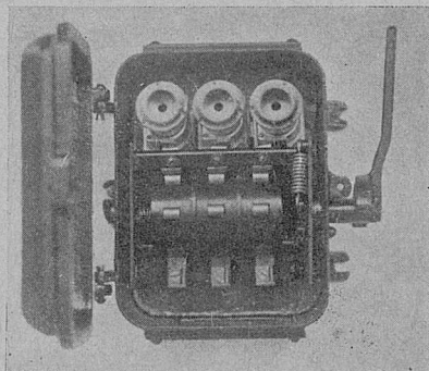
Skrzynki przyłączowe, gwiazda — trójkąt i prze- łączniki kierunku obrotu
