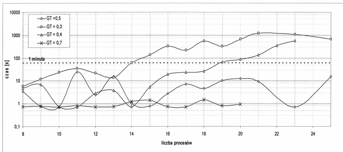
Rys. 5.17. Zależność czasu wyznaczania pierwszego warunku wystarczającego od liczby procesów realizowanych w systemie transportowym
