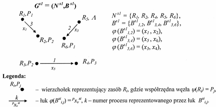
Rys. 4.13. Przykładowa postać grafu nie zawierającego żadnego podgrafu {}^zG^{si}
