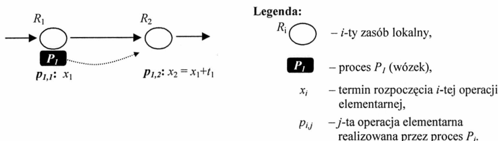
Rys. 4.7. Obsługa procesu przez zasoby lokalne
