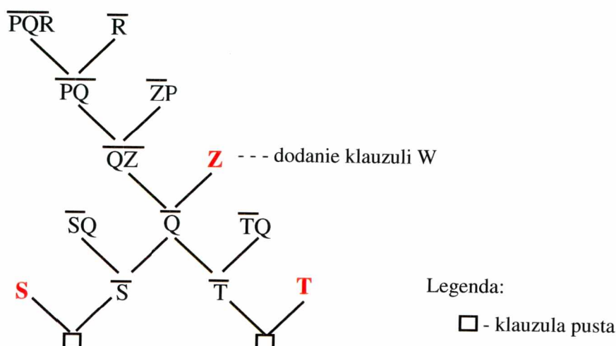
Rys. 3.3. Drzewo rezolucji
