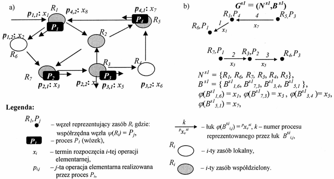
Rys. 4.14. Przykład stanu systemu SWPC: a) stan S_1 , b) graf G^{s1}
