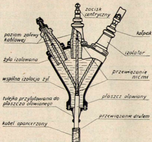
Rys. 4. Głowica płaska.
