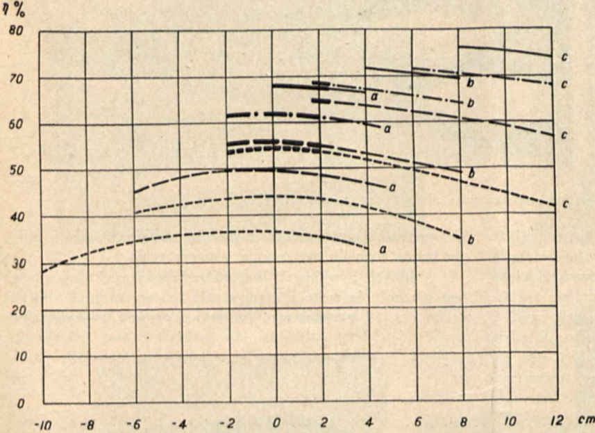
Rys. 3. Sprawności przygotowania różnej ilości wody na płytkach różnych średnic. 1 litr - - - - - 2 litry - - - - - 4 litry - - - - - 6 litrów - - - - - a - na płytce \phi 22 cm, b - na płytce \phi 18 cm, c - na płytce \phi 14,5 cm.
