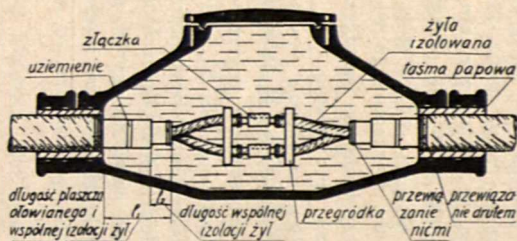
Rys. 5. Mufa złączowa.
