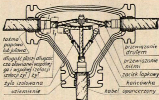
Rys. 6. Mufa odgałęznej do nieprzecinanego kabla wielożyłowego.
