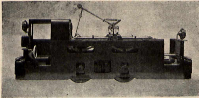
Rys. 4. Lokomotywa kopalniana zaopatrzona w 2 silniki trakcyjne o mocy godzinowej 23 kW, 660 obr./min. (Rohn-Zieliński S. A.).
