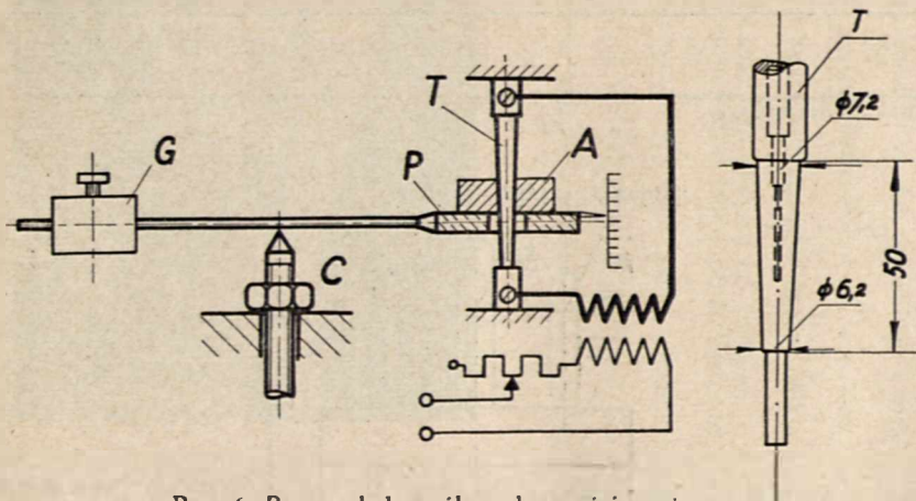
Rys. 6. Przyrząd do próby odporności na żar
