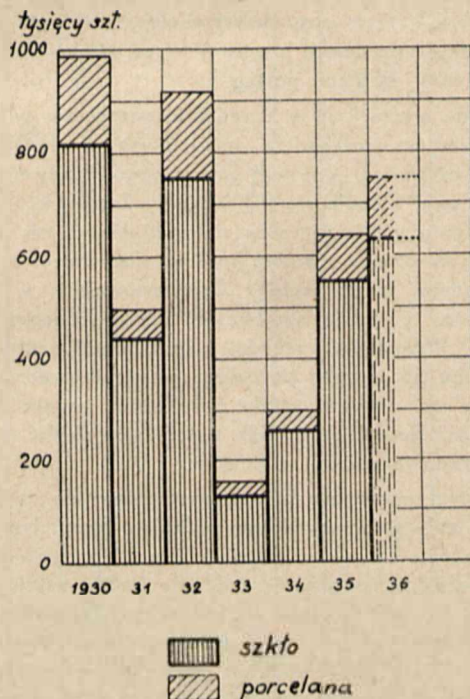
Rys. 4. Zapotrzebowanie izolatorów teletechnicznych przez M. P. i T. oraz M. K.
