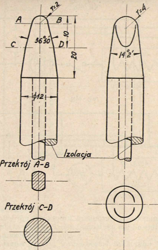
Rys. 1. Palec probierczy.
