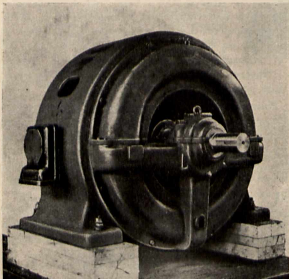
Rys. 5. Trójfazowy silnik asynchroniczny. 315 KM, 5000 V, 330 obr./min. (Rohn-Zieliński S. A.).
