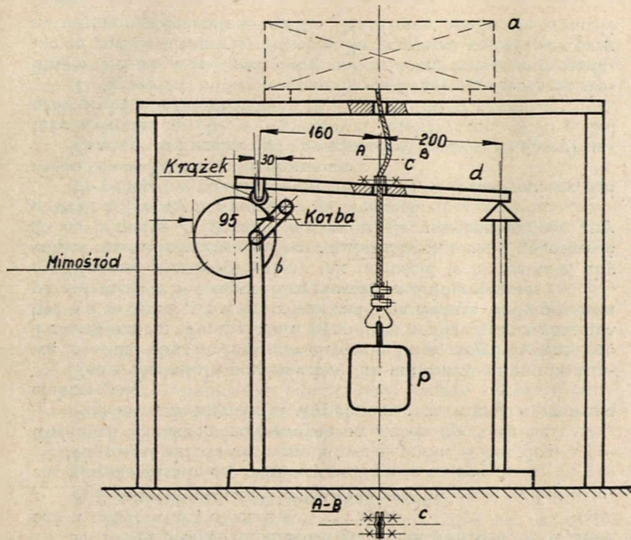
Rys. 4. Przyrząd do próby zamocowania przewodu w grzejniku.
