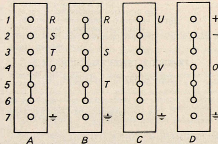
Rys. 8. Schemat połączeń zacisków kuchen z piekarnikami.
