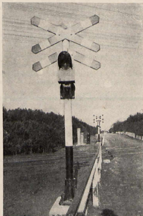
Rys. 16. Sygnalizacja na przejeździe kolejowym.
