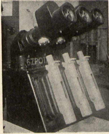
Fot. 5. Wyłącznik powietrzny bezsprężarkowy typu 603.
