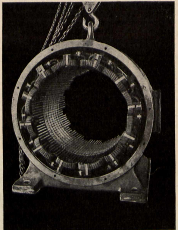
Rys. 6. Stojan trójfazowego silnika asynchronicznego 280 KM, 2000 V. (Rohn-Zieliński S. A.).
