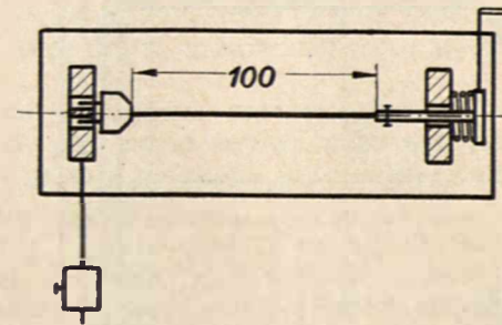
Rys. 5. Przyrząd do próby zabezpieczenia przed skręceniem żył
