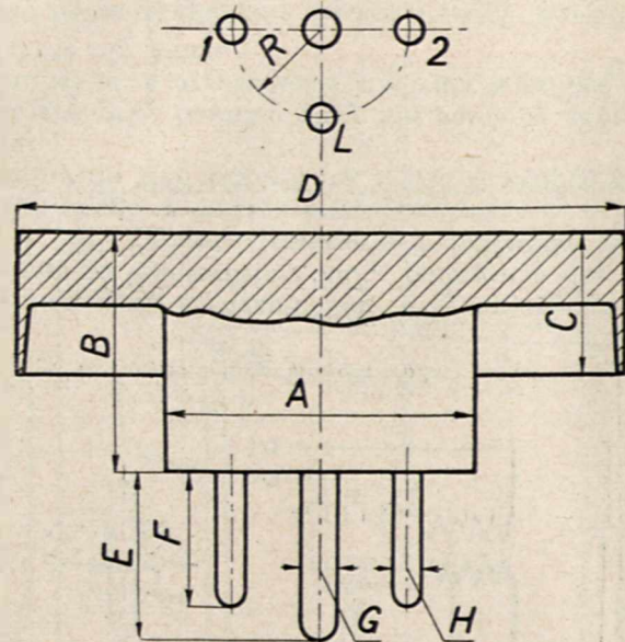
Rys. 7. Wymiary płytki grzejnej.
