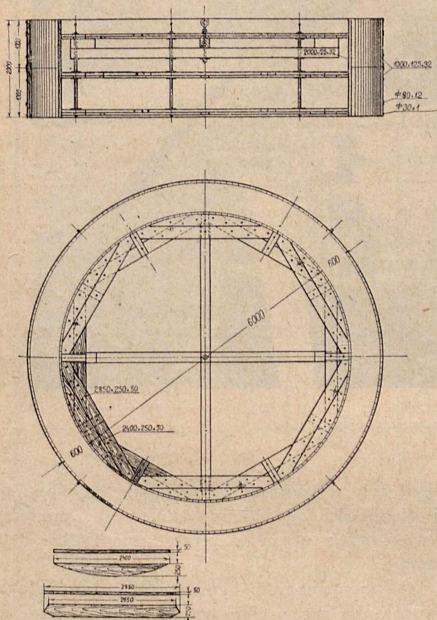
Rys. 8. Deskowanie.
