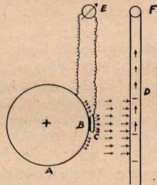
Rys. 1. Elektroda pomocnicza dla pomiarów prądów błędnych. A — rura, B — izolacja asfaltowa, C — elektroda pomocnicza, D — przewód powrotny tramwaju, E — amperomierz, F — punkt zasilania.
