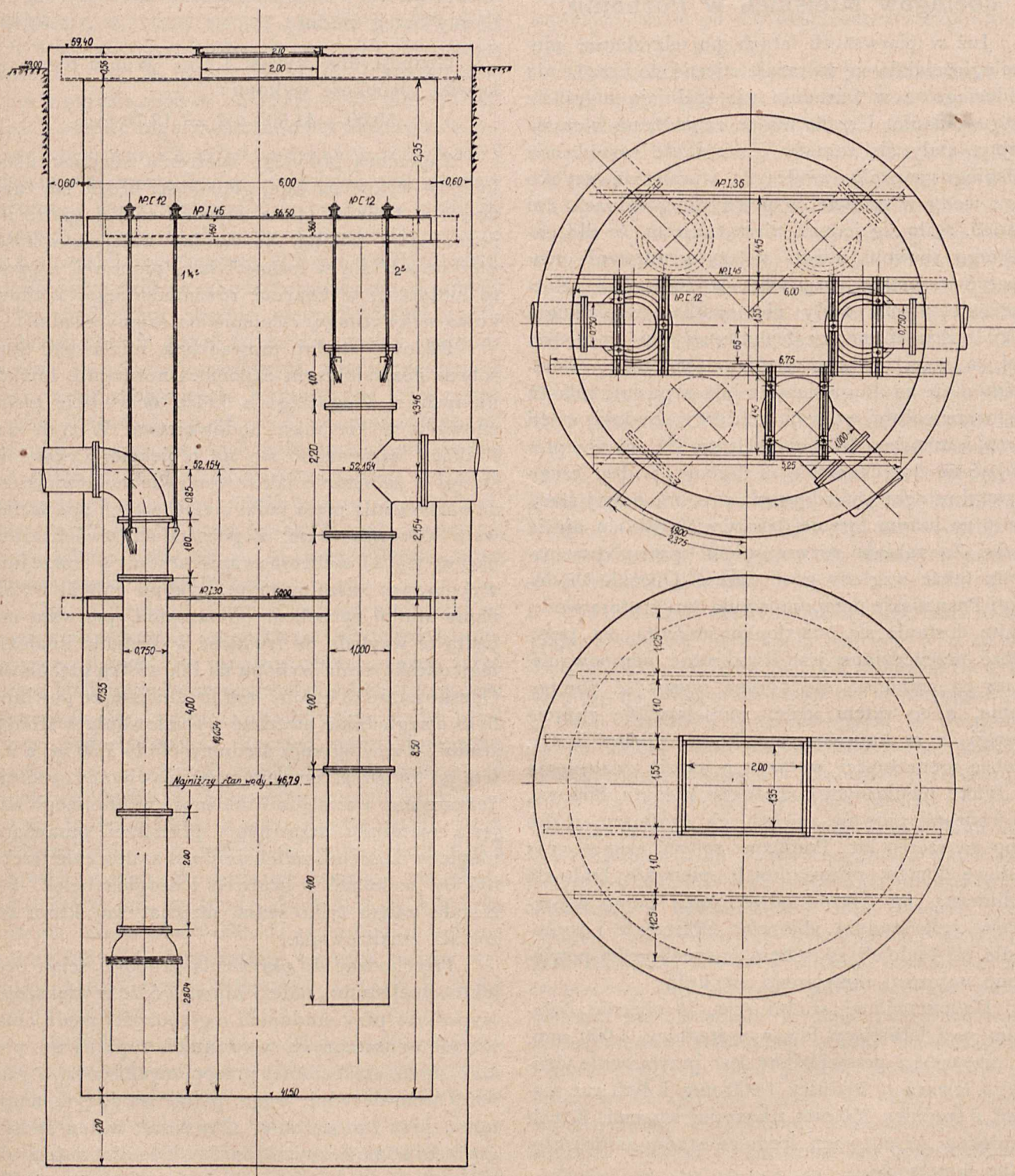
Rys. 1. Studnia zbiorcza.
