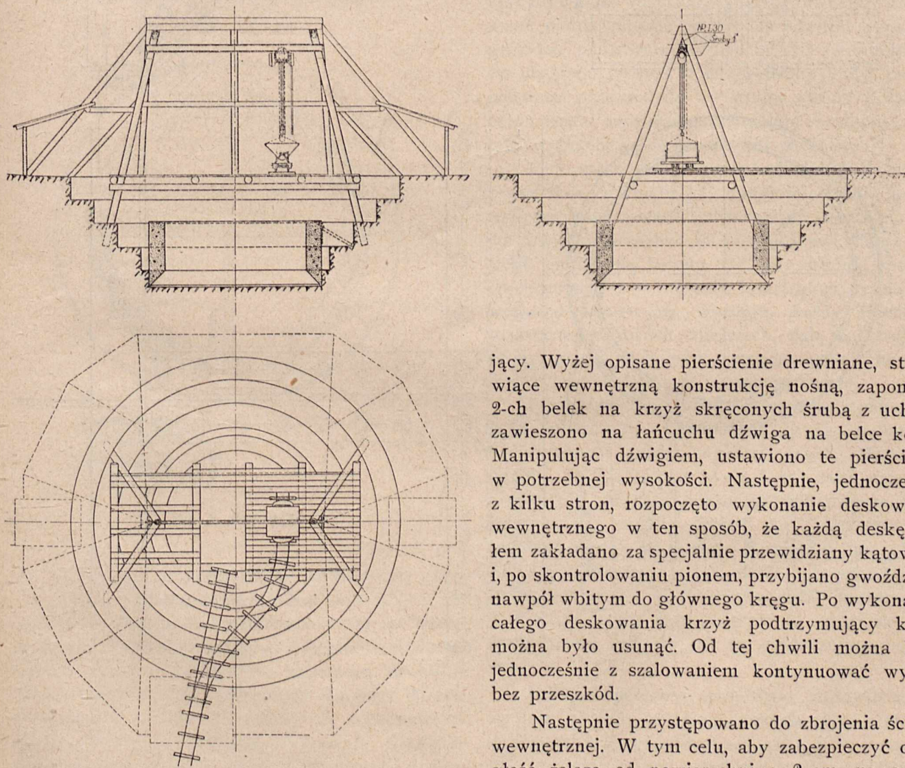
Rys. 6. Wykop i kocioł.
