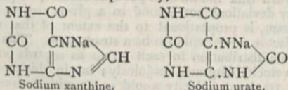
Sodium xanthine.
