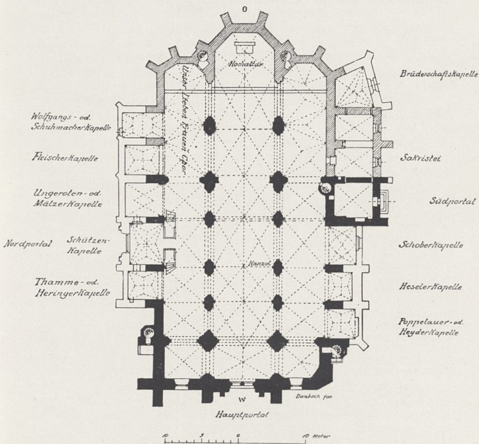
Grundriss der Peter-Paul-Kirche zu Liegnitz im Mittelalter.
