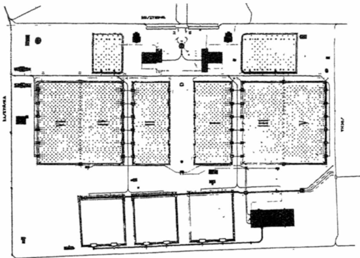
Rys. 3. Plan Stacji Filtrów.
