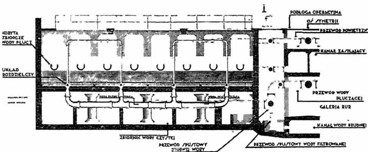
Rys. 4. Przekrój poprzeczny hali filtrów w Zakładzie Filtrów Pośpiesznych.
