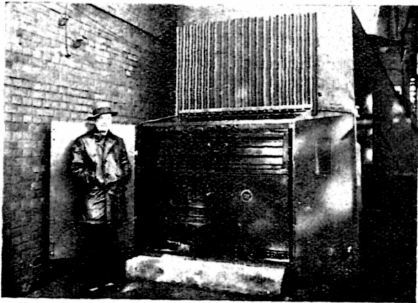
Rys. 1. Automacyjny regulator Aeosolo, zainstalowany u podnóża kominu w Gazowni Miejskiej w Bydgoszczy.
