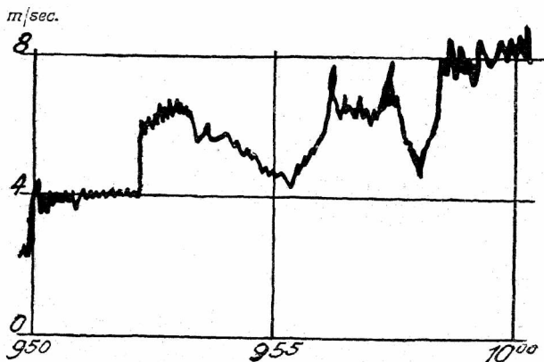
Rys. 2 a. Wahania siły wiatru przy słabym wietrze.
