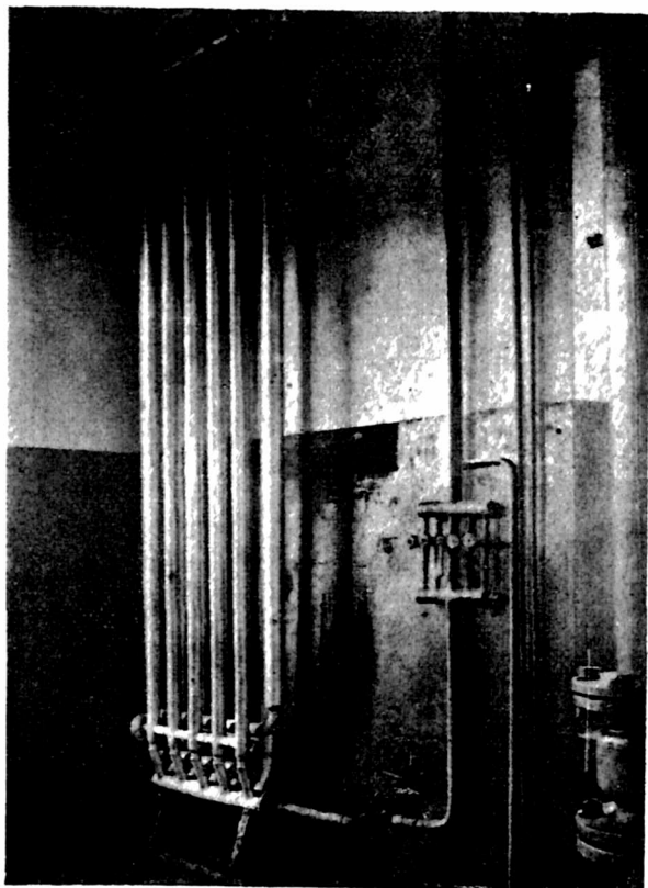
Rys. 3 Podgrzewacz gazu (z prawej strony widoczny zawór ekspansyjny).
