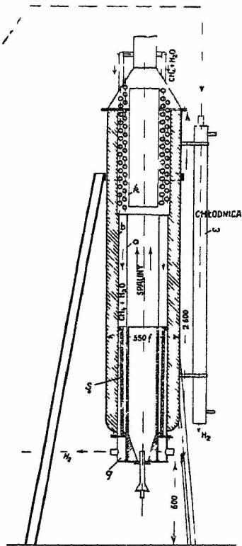
Rys. 3. Generator doświadczalny do przeróbki gazu ziemnego z parą wodną na wodór.
