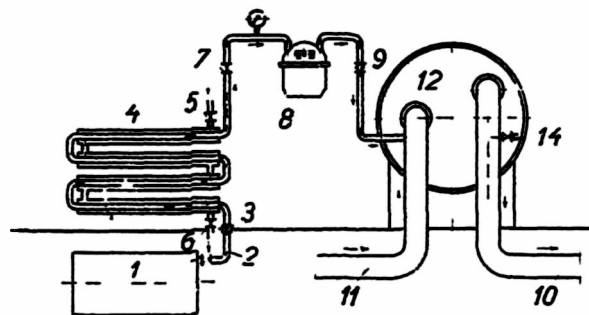
Rys. 1. Aparatura prowizoryczna dla produkcji gazu gazolowo-powietrznego.
