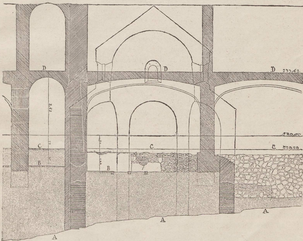
AAA-skala, BBB -posadzka renesansowa, CCC-posadzka austriacka, DDD-posadzka austriacka pierwszego piętra. Stan po wykopaliskach, dokonanych w latach 1911-12
