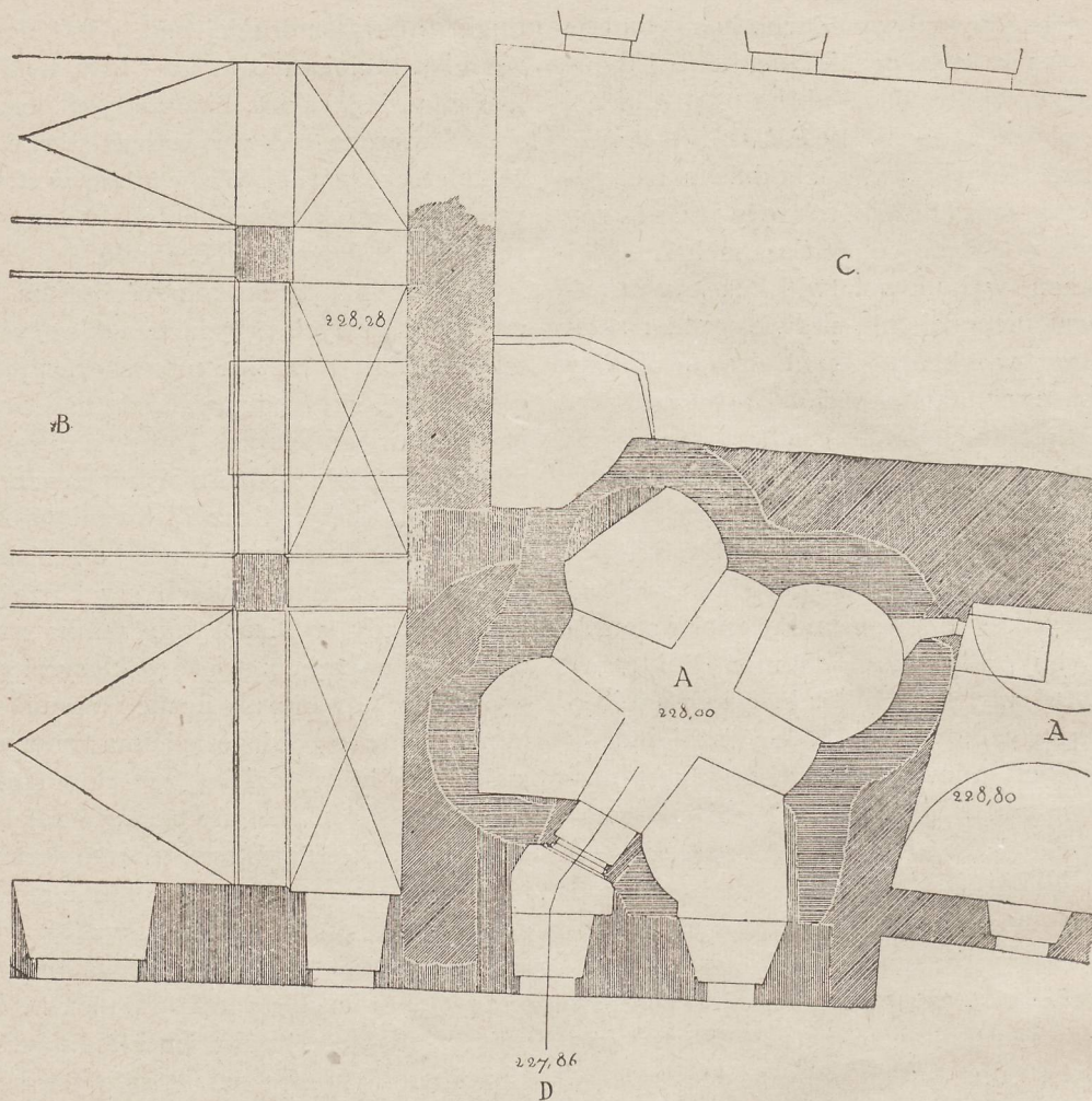
— Mur pierwotny, // mur gotycki, ||| mur renesansowy Przekroju murów dokonano na wysokości 229,00 od powierzchni wody w oceanie AA—mieszkanie podrzędne, B Kuchnie królewskie, C—podwórczyk gospodarczy, D—podwórcze arkadowy zamkowy
