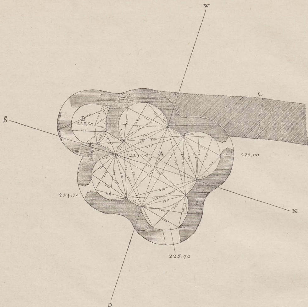
— Mur pierwotny, // mur gotycki 1241 r. Przekroju murów dokonano na wysokości 226,65 nad powierzchnią oceanu. A - kościół, B - zakrystya, C - mur obronny XIII w. Kreskowanie rozrzedzone oznacza mur już nieistniejący
