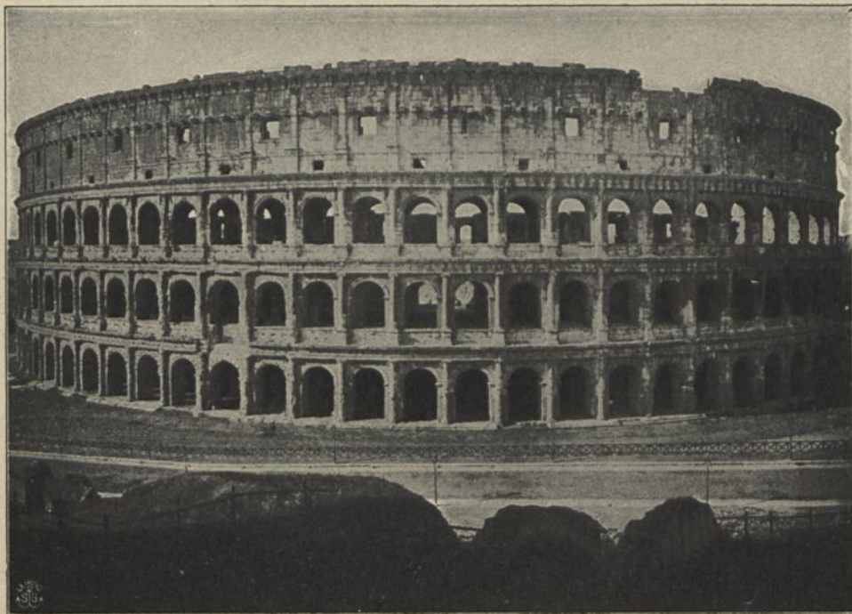
Fig. 105. Kolosseum. Rzym.
