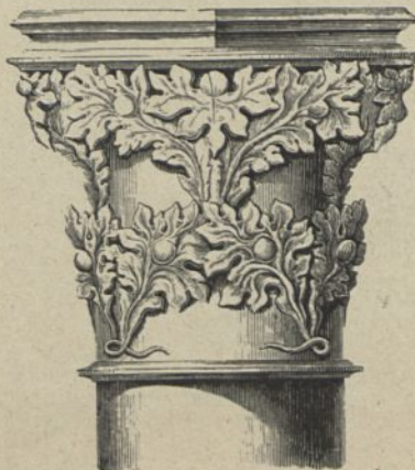
Fig. 144. Kapitel gotycki.
