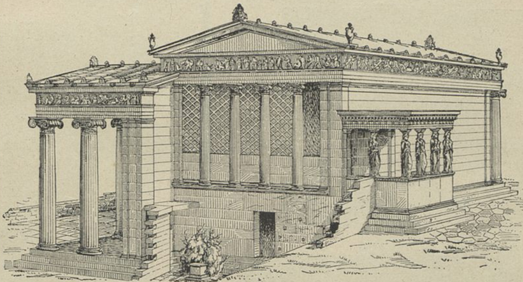
Fig. 27. Erechtheion. Atheny.
