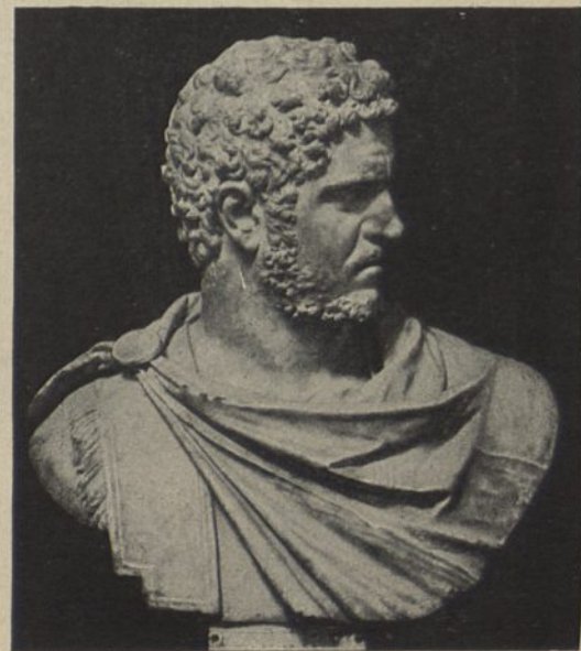
Fig. 103. Caracalla. Neapol.
