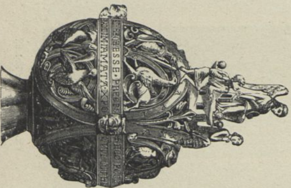
Fig. 188. Kadzielnica romańska.
