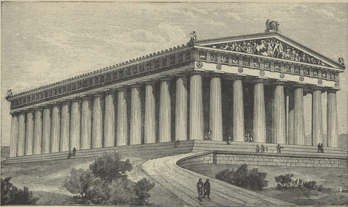
Fig. 26. Parthenon. Atheny.
