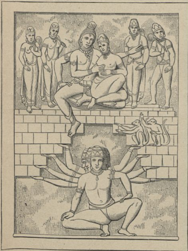
Fig. 10. Świątynia Ellory.
