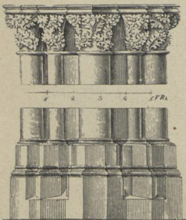
Fig. 143. Stup gotycki.
