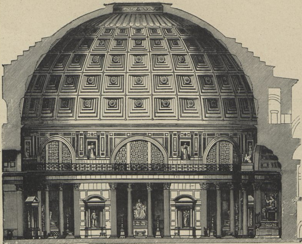
Fig. 104. Pantheon. Rzym.
