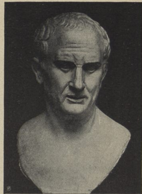
Fig. 102. Cicero. Londyn.
