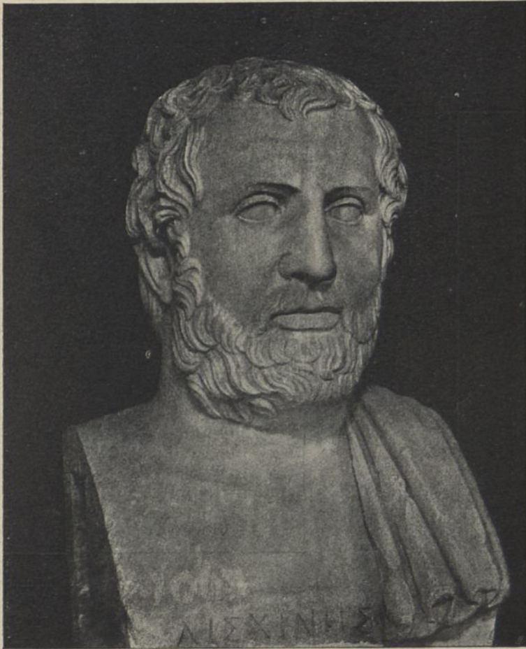
Fig. 82. Aeschynes. Vatykan.
