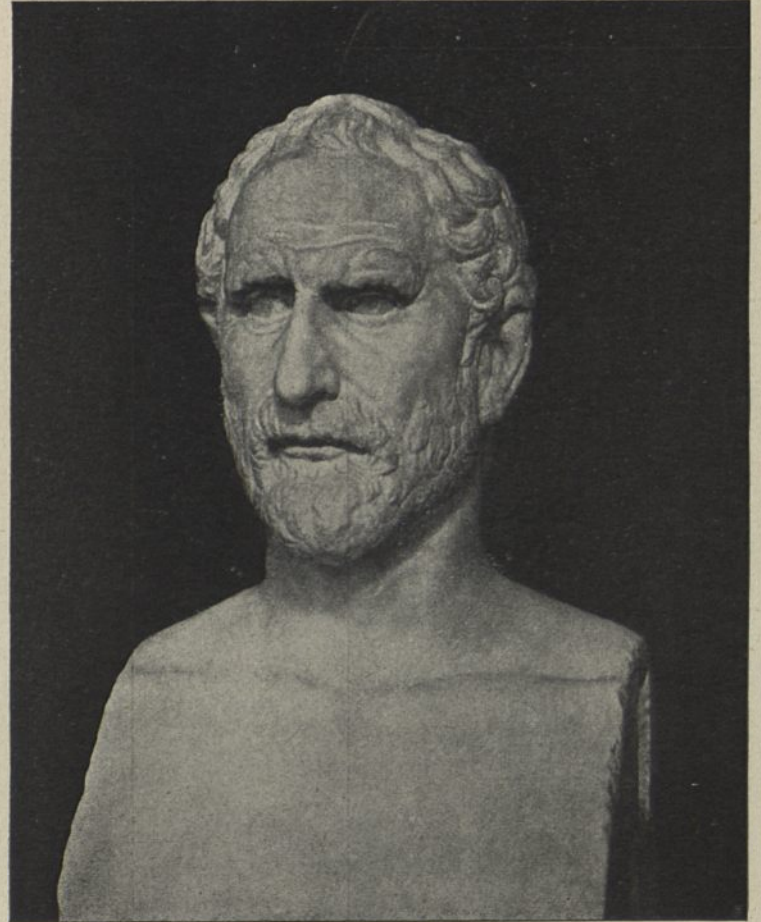
Fig. 83. Demostenes. Vatykan.
