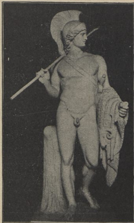
Fig. 364. Thorwaldsen. Jason.
