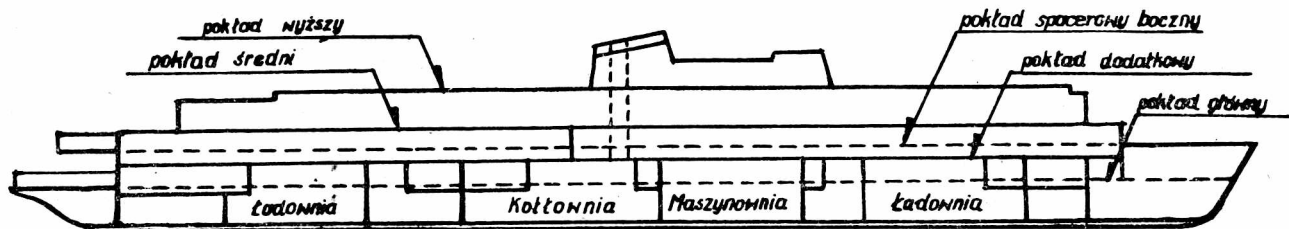
rys. 1 Schematyczny zład podłużny z widocznymi różnicami poziomów z zewnątrz i wewnątrz nadbudówek.
