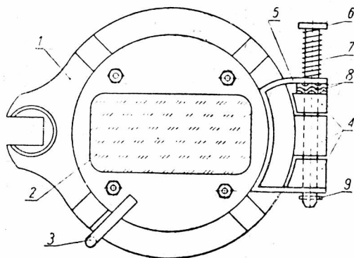
Rys. 4. Oprawa szkła ochronnego: 1 — oprawa szkła ochronnego, 2 — szkło ochronne, 3 — rączka, 4 — zawiasy, 5 — zawiasa dodatkowa, 6 — trzpień mosiężny, 7 — sprężyna, 8 — podkładki sześciokątne przylutowane do zawiasów, 9 — zatyczka.
