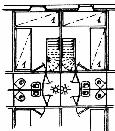
rys. 3 Nowy układ kabin: apartament na dwóch poziomach z własnym balkonem, wychodzącym na boczny pokład spacerowy
