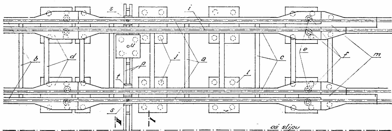
Rys. 2. Rzut poziomy
