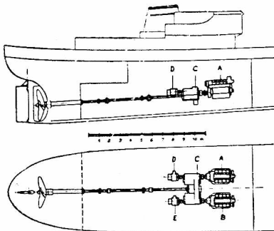
Rys. 2. Napęd trawlera BELGIAN SKIPPER. A i B — silniki główne; C — przekładnia wielostopniowa; D i E — prądnice do napędu windy trawlowej i mechanizmów pomocniczych.
