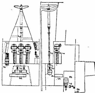
Rys. 3. Siłownia trawlera z napędem diesel-elektrycznym. 1 — główne zespoły prądotwórcze (silnik prądnica); 2 — wał śrubowy; 3 — przekładnia silników napędowych śruby; 4 — silniki napędowe śruby; 5 — główna tablica rozdzielcza; 6 — silnik windy trawlowej; 7 — urządzenie regulacyjne windy trawlowej; 8 — stanowisko manewrowe (mostek); 9 — pomocniczy zespół prądotwórczy.
