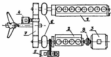
Rys. 1. Schemat napędu „Ojciec i syn”. 1 — 8-cylindrowy silnik napędowy, nawrotny; 2 — 4-cylindrowy silnik napędowy śruby i windy trawlowej, nienawrotny; 3 — prądnica i windy trawlowej; 4 — prądnica z napędem od układu głównego; 5 — zespół prądnica-sprężarka; 6 — sprzęgła hydrauliczne; 7 — przekładnia mechaniczna; 8 — sprzęgło rozłączne.
