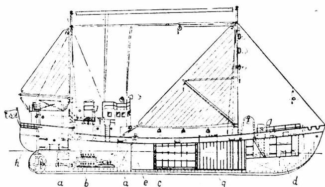
Rys. 2. SRT — średni trawler rybacki, w zasadzie lugier, mogący trawlować. a — paliwo; b — silnik główny; c — izolacja; d — balast; e — sieci i liny; f — ładownia na ryby w lodzie; g — ładownia na beczki; h — prowiant.
