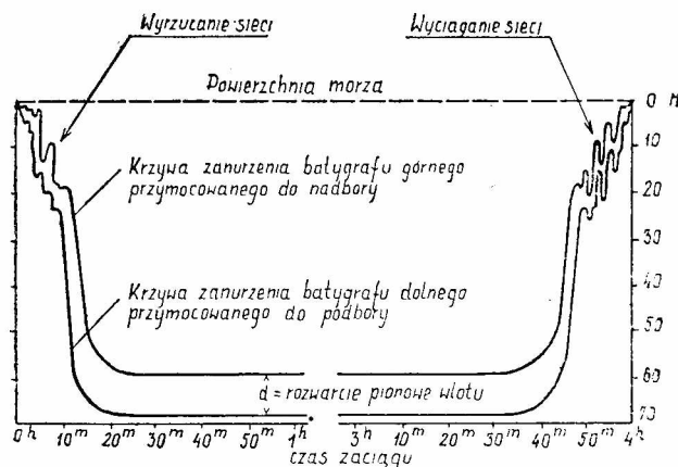
Rys. 1. Zestawienie 2 batygrafów tj. wykresów 2 batygrafów przymocowanych do nadbory i podbory.
