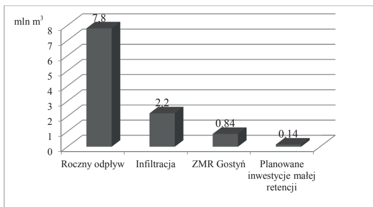
Rys. 2. Porównanie potencjalnych efektów zabiegów nietechnicznych i technicznych (projektowany ZMR Gostyń oraz planowane w programie małej retencji budowle piętrzące i stawy) oraz średniego rocznego odpływu ze zlewni rzeki Kania
