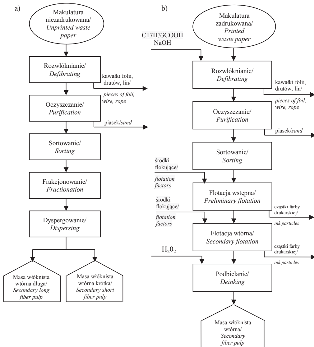
Rys. 3. Schemat ideowy przerobu makulatury:
